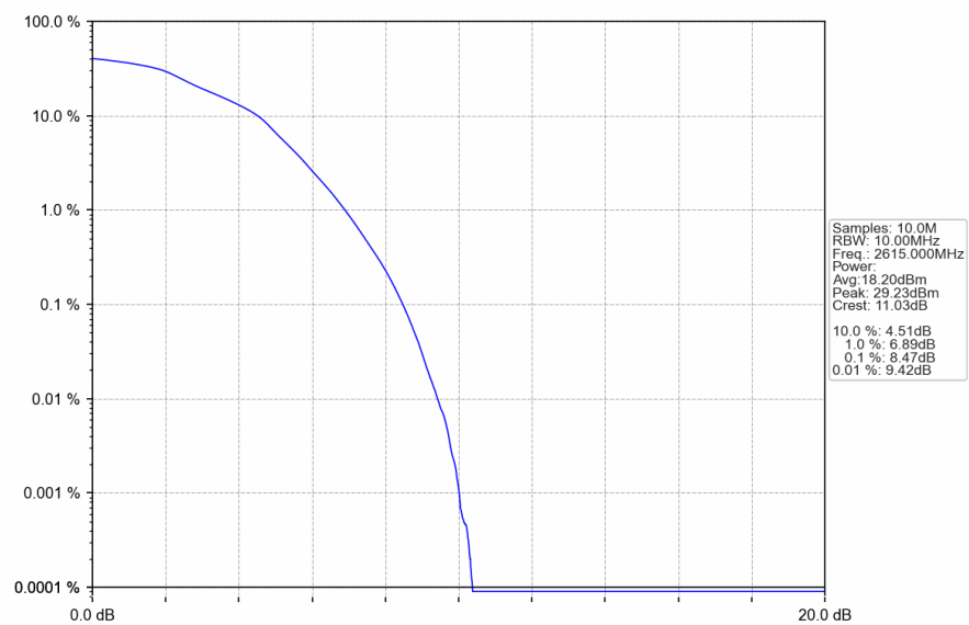
Band38 10MHz 16QAM HCH 2615MHz RB 50 0 NTNV
