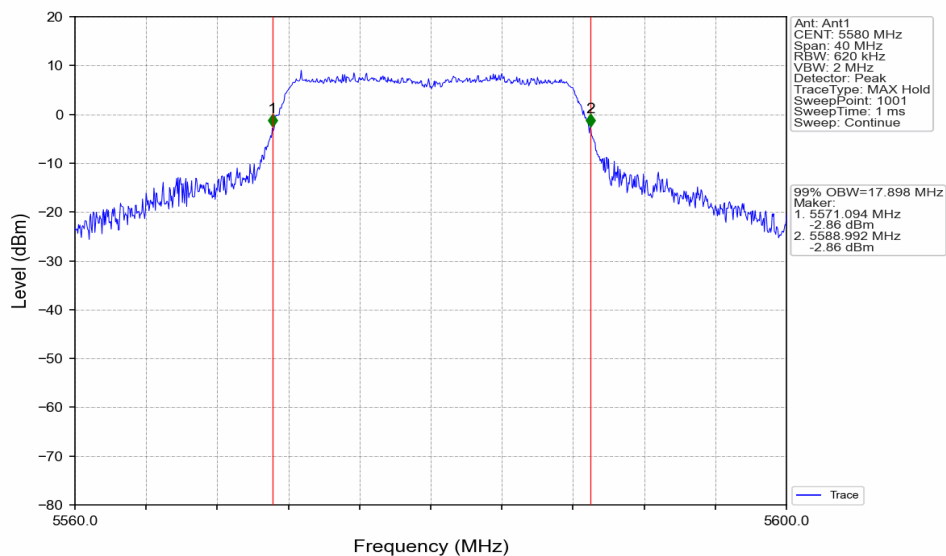
802.11a_MCH_5580MHz_Ant1_NTNV
