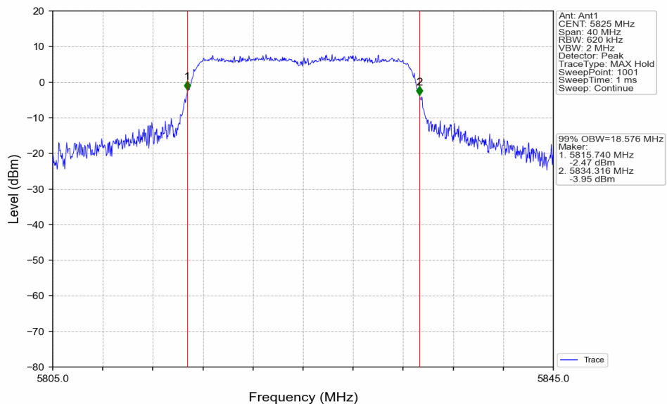
802.11n(HT20)_HCH_5825MHz_Ant1_NTNV
