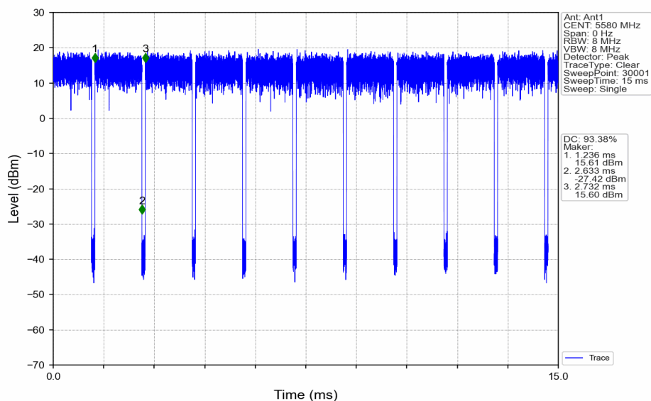
802.11a_MCH_5580MHz_Ant1_NTNV
