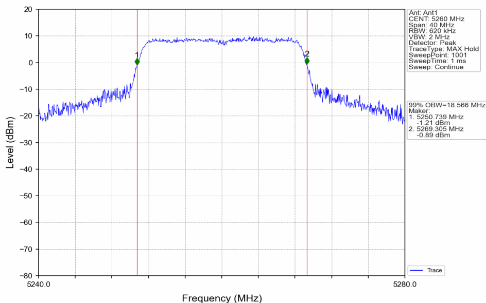
802.11n(HT20)_LCH_5260MHz_Ant1_NTNV
