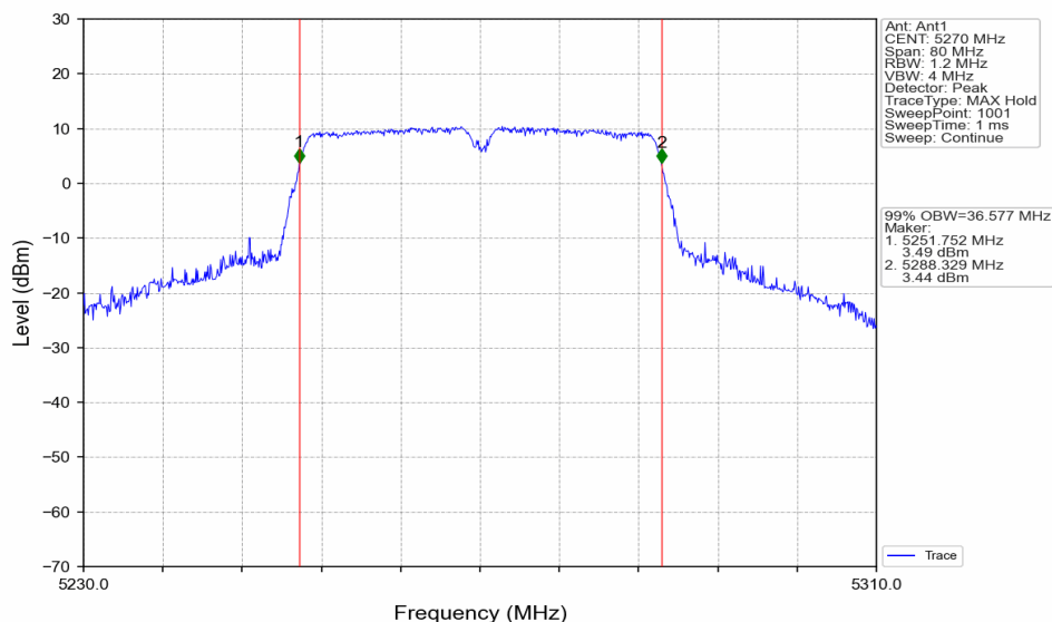
802.11ac(VHT40)_LCH_5270MHz_Ant1_NTNV
