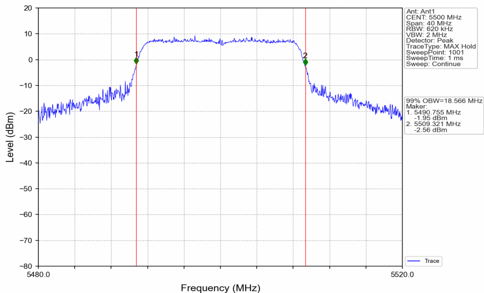
802.11ac(VHT20)_LCH_5500MHz_Ant1_NTNV
