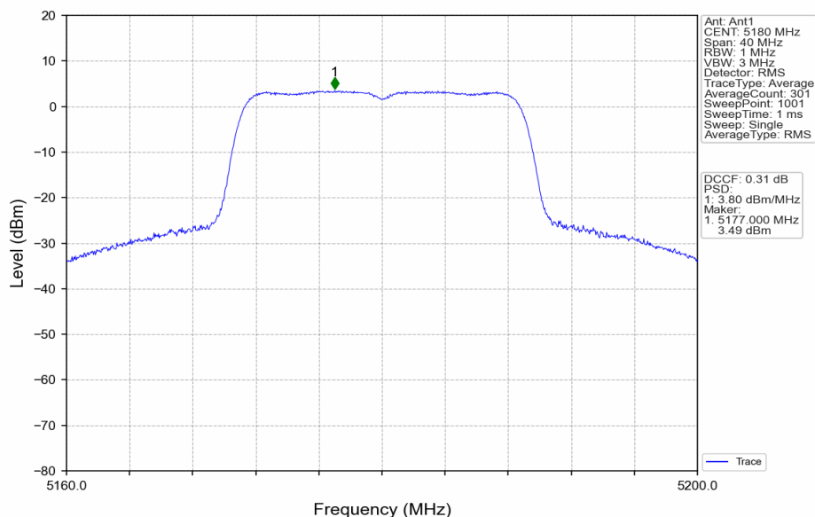
802.11n(HT20)_LCH_5180MHz_Ant1_NTNV
