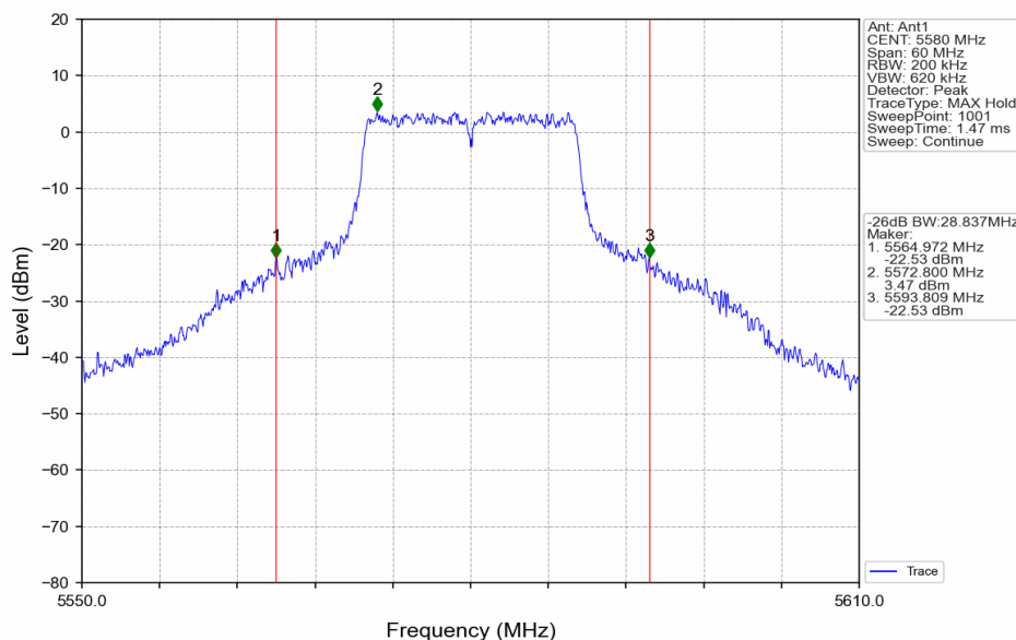
802.11a_MCH_5580MHz_Ant1_NTNV
