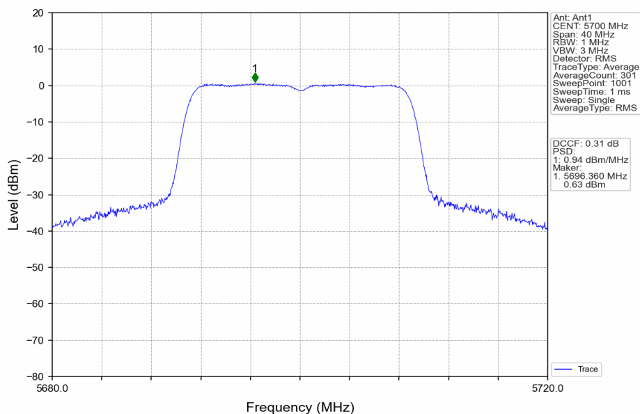
802.11ac(VHT20)_HCH_5700MHz_Ant1_NTNV
