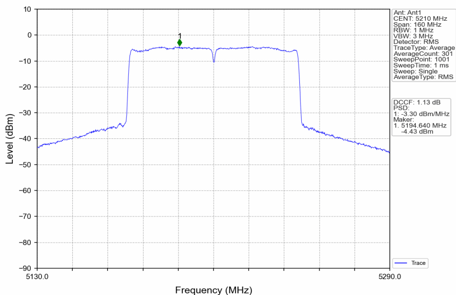
802.11ac(VHT80)_MCH_5210MHz_Ant1_NTNV
