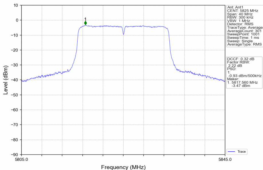
802.11n(HT20)_HCH_5825MHz_Ant1_NTNV
