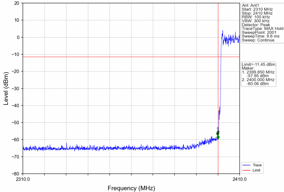
Pi/4DQPSK_2DH5_HOPP_Ant1_NTNV
