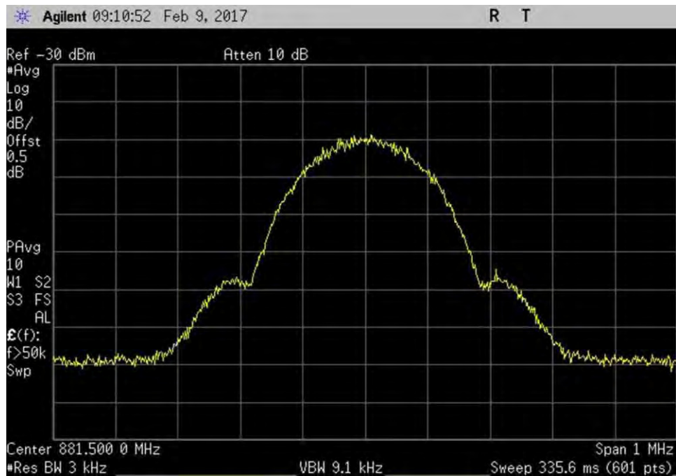
7.10_OBW_DL_869-894MHz_GSM_In
