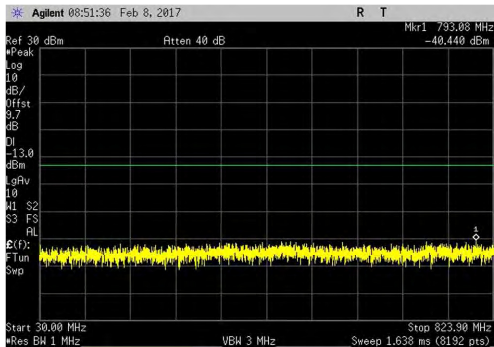
7.6_CSE_UL_824-849MHz_L
