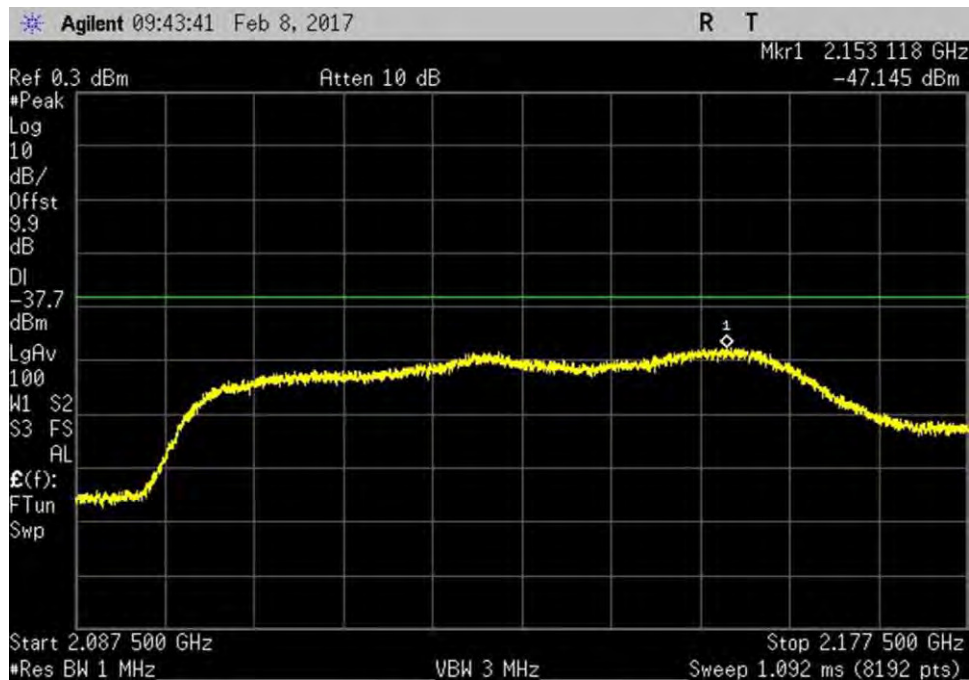
7.7.1_Noise_DL_2110-2155MHz
