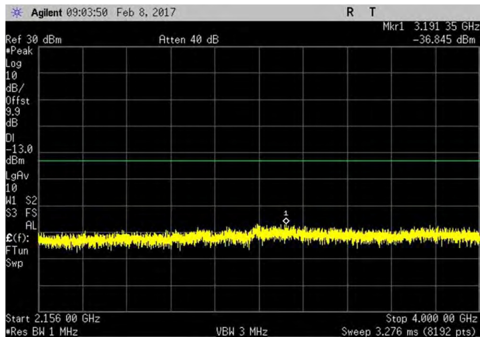
7.6_CSE_DL_2110-2155MHz_R1
