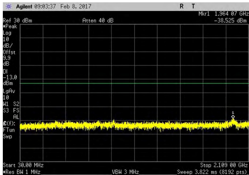
7.6_CSE_DL_2110-2155MHz_L
