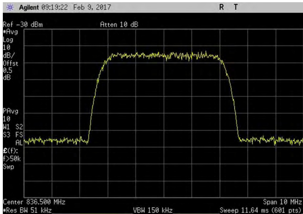
7.10_OBW_UL_824-849MHz_WCDMA_In
