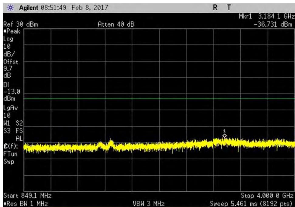
7.6_CSE_UL_824-849MHz_R1
