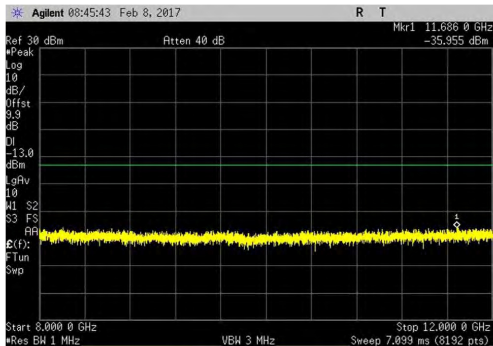
7.6_CSE_UL_1710-1755MHz_R3
