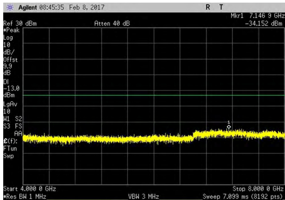
7.6_CSE_UL_1710-1755MHz_R2
