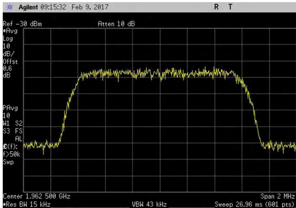
7.10_OBW_DL_1930-1995MHz_CDMA_In
