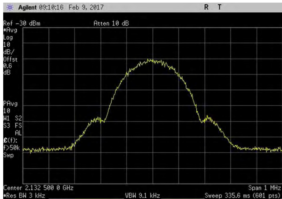
7.10_OBW_DL_2110-2155MHz_GSM_In
