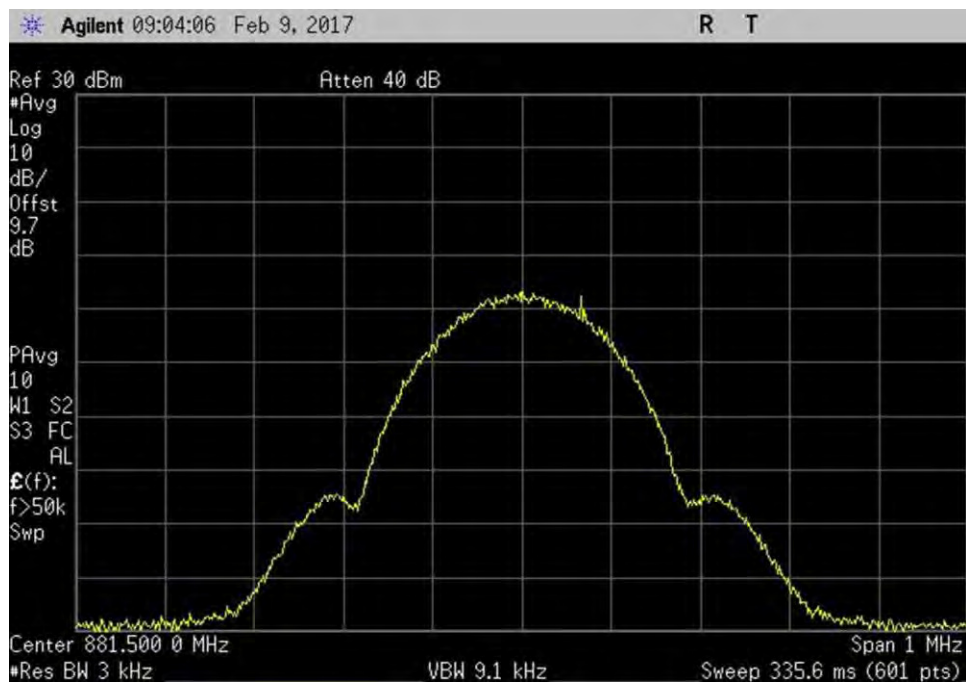
7.10_OBW_DL_869-894MHz_GSM_Out
