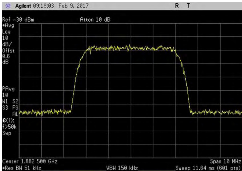
7.10_OBW_UL_1850-1915MHz_WCDMA_In
