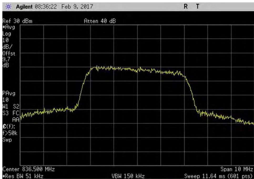
7.10_OBW_UL_824-849MHz_WCDMA_Out
