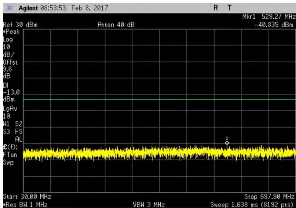
7.6_CSE_UL_698-716MHz_L
