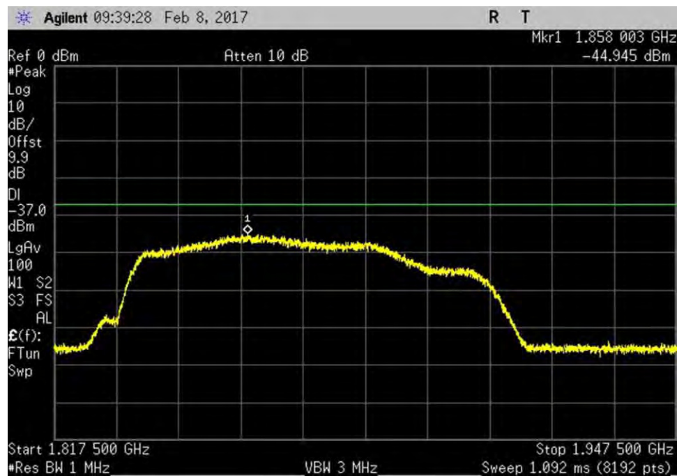
7.7.1_Noise_UL_1850-1915MHz
