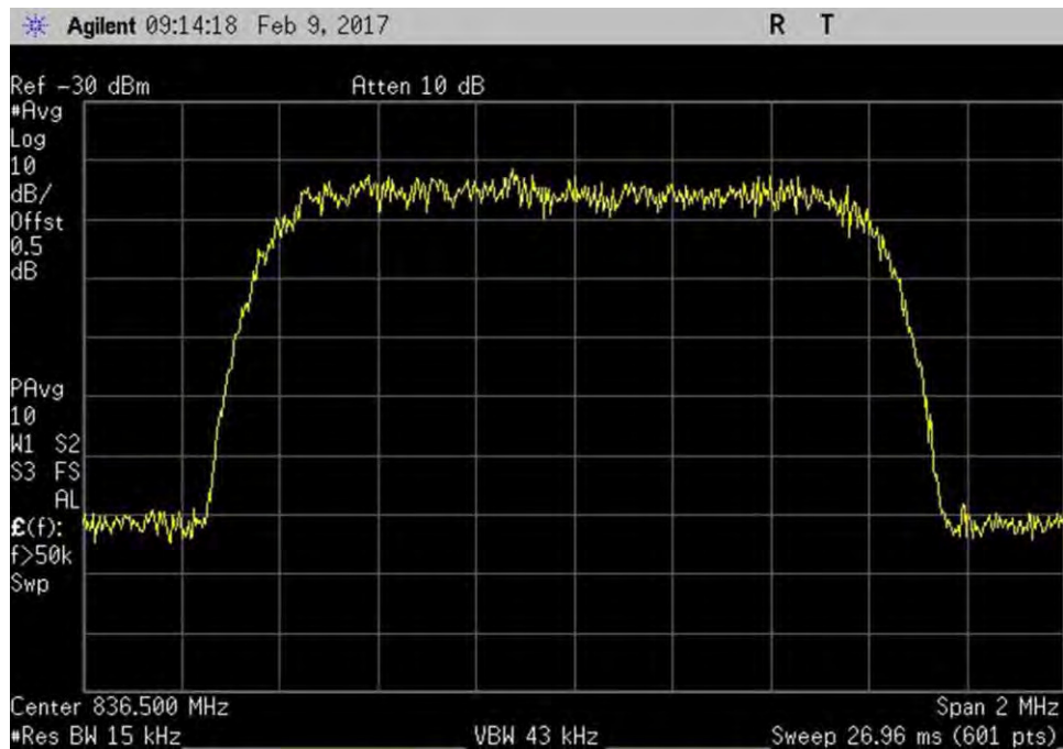
7.10_OBW_UL_824-849MHz_CDMA_In
