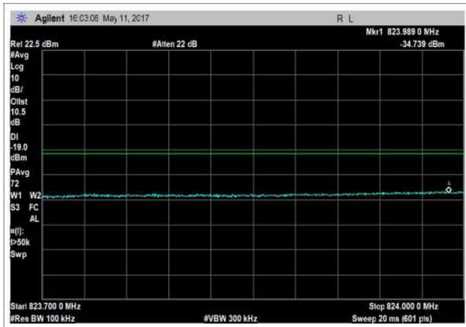
UL_824-849MHz_L_PreAGC_CDMA
