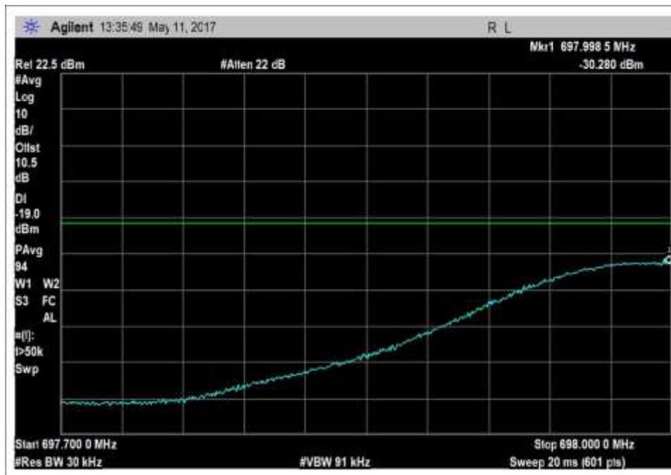
UL_698-716MHz _L_PreAGC_GSM
