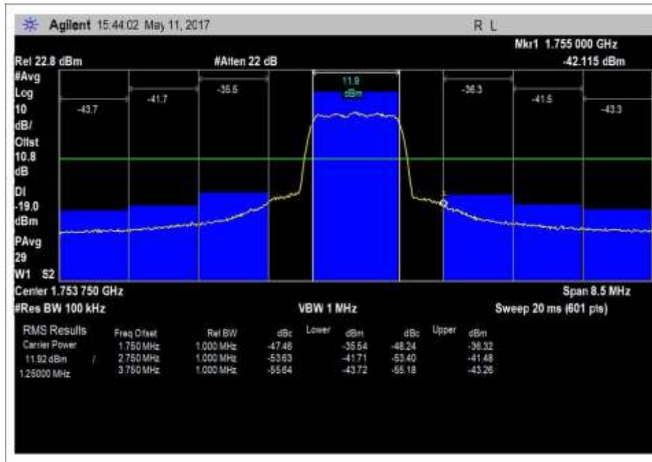
UL_1710-1755MHz_H_PreAGC_CDMA
