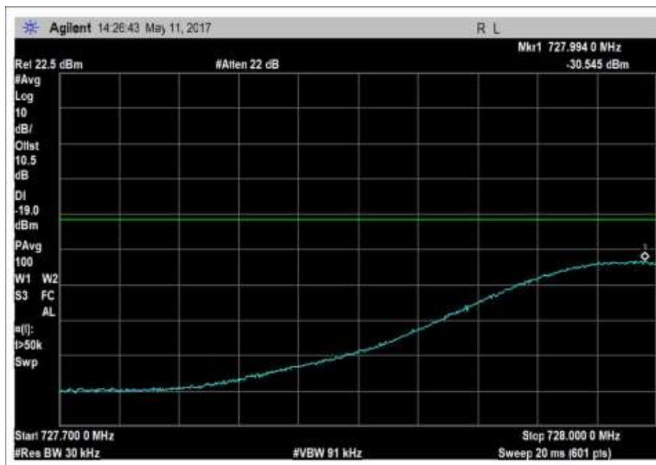
DL_728-746MHz _L_PreAGC_GSM
