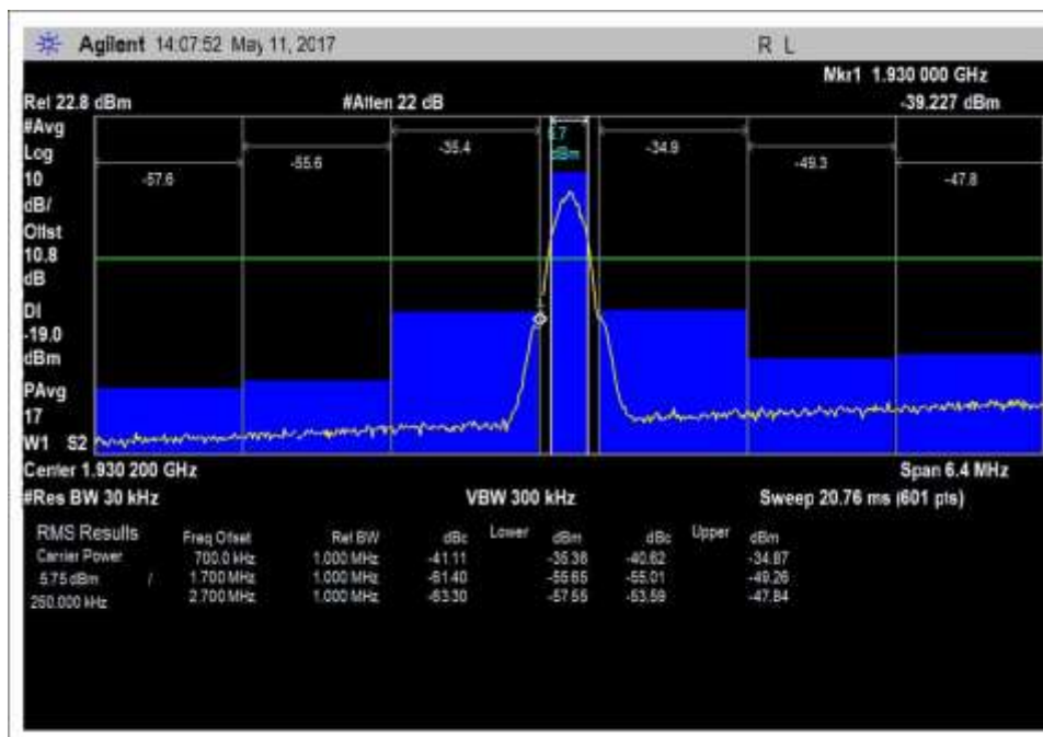
DL_1930-1995MHz _L_PreAGC_GSM
