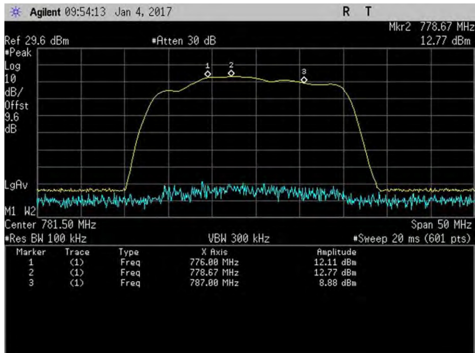
7.1_Band Verify_UL_776-787MHz_Zoom
