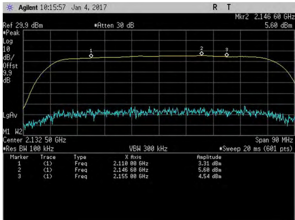
7.1_Band Verify_DL_2110-2155MHz
