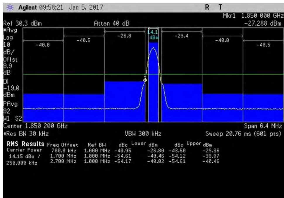
7.5_OBE_UL_1850-1915MHz_L_PreAGC_GSM
