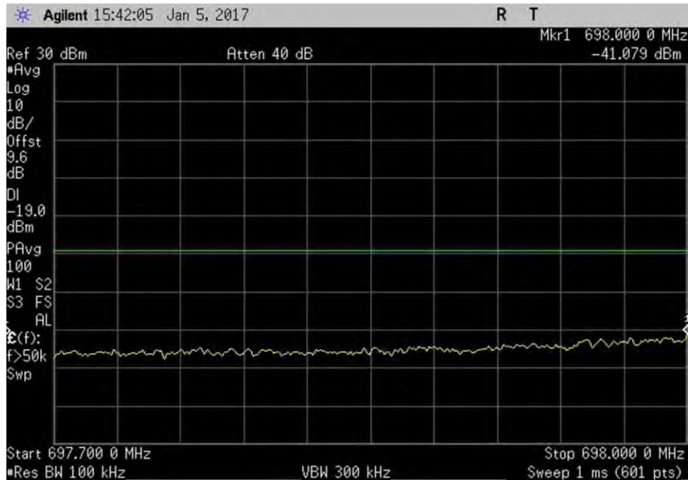
7.5_OBE_UL_698-716MHz_L_PreAGC_LTE
