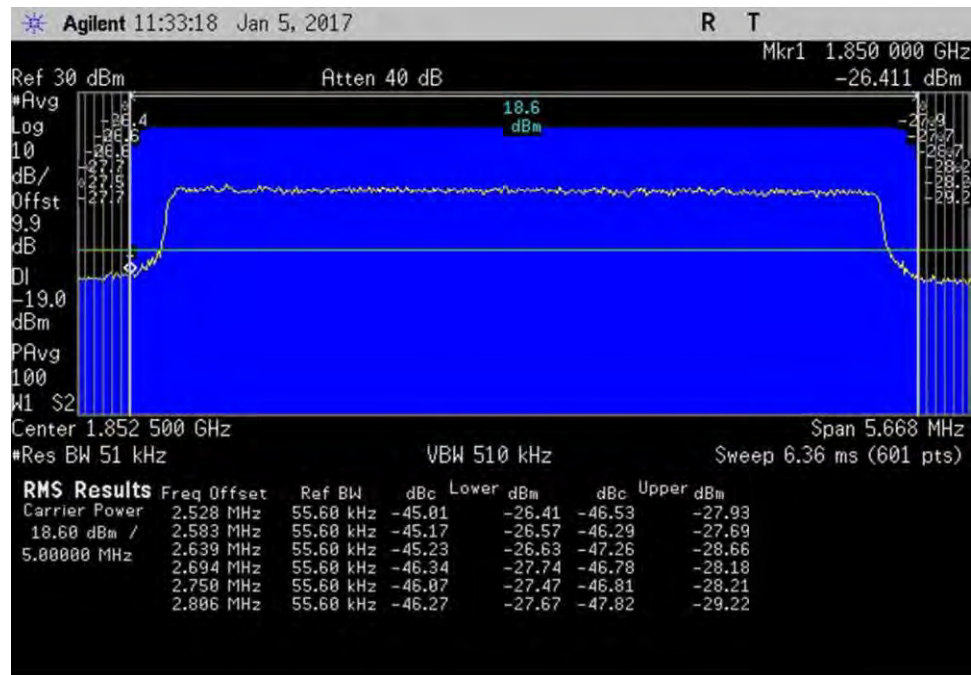
7.5_OBE_UL_1850-1915MHz_L_PreAGC_LTE
