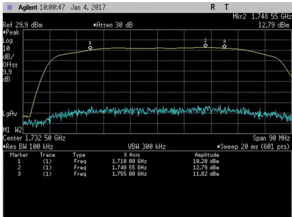
7.1_Band Verify_UL_1710-1755MHz
