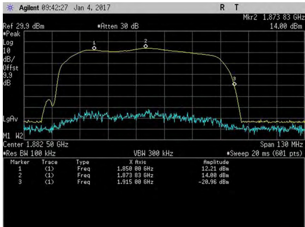
7.1_Band Verify_UL_1850-1915MHz
