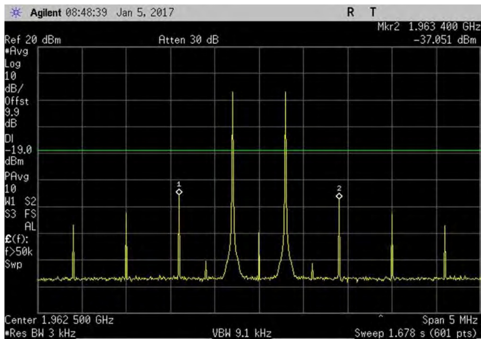
7.4_Intermod_DL_1930-1995MHz
