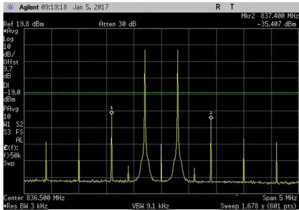
7.4_Intermod_UL_824-849MHz
