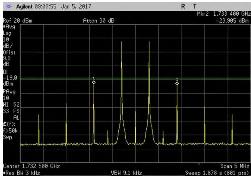
7.4_Intermod_UL_1710-1755MHz
