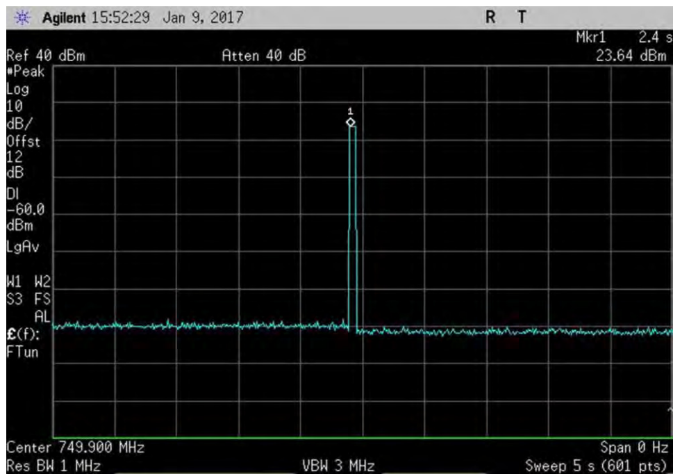
7.11.2_osc_DL_746-757MHzPk
