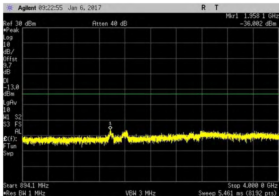
7.6_CSE_DL_869-894MHz_R1
