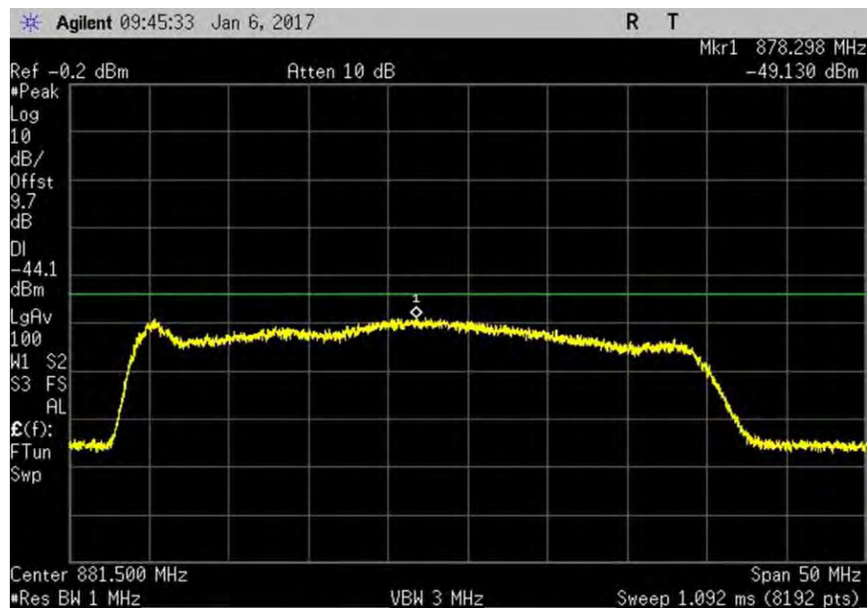
7.7.1_Noise_DL_869-894MHz
