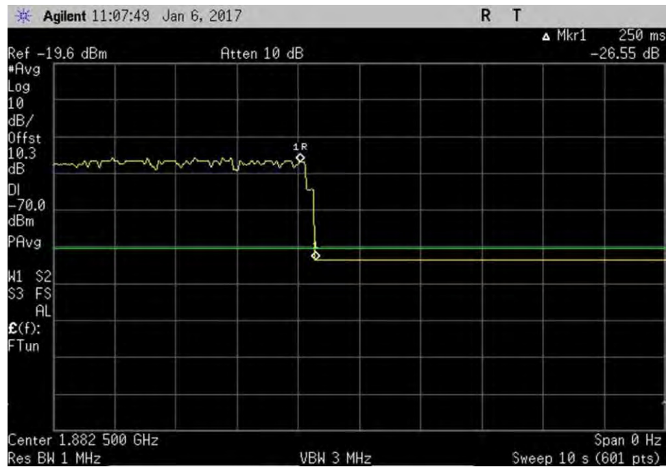
7.7.2_VarNoise_UL_1850-1915MHz
