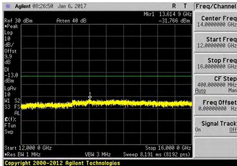
7.6_CSE_UL_1710-1755MHz_R4
