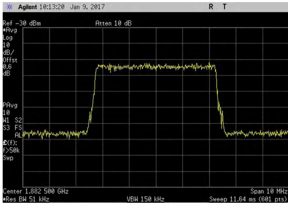
7.10_OBW_UL_1850-1915MHz_LTE_In
