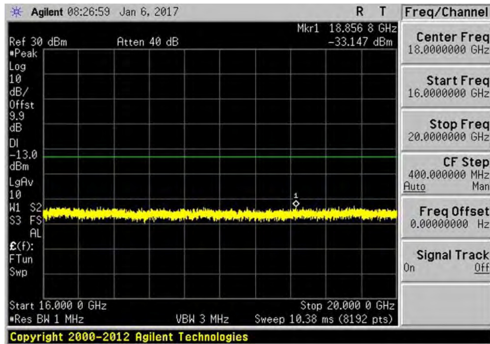
7.6_CSE_UL_1710-1755MHz_R5
