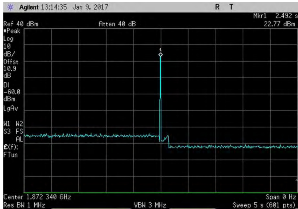
7.11.2_osc_UL_1850-1915MHzPk
