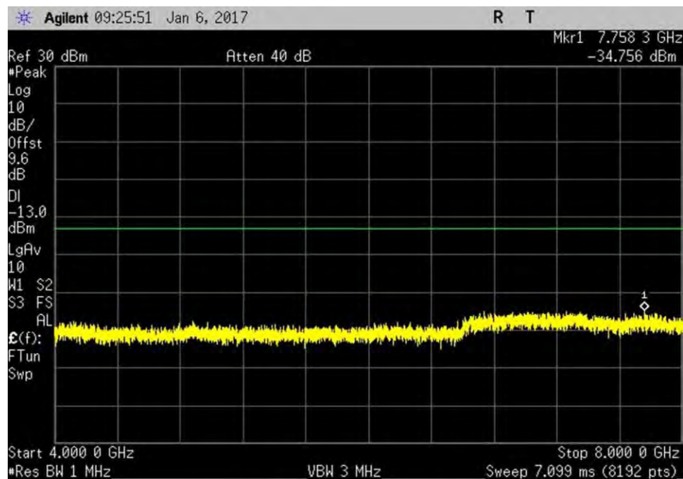
7.6_CSE_DL_728-746MHz_R2
