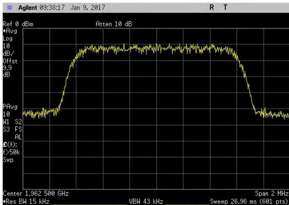
7.10_OBW_DL_1930-1995MHz_CDMA_Out
