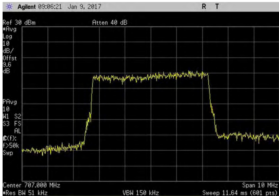
7.10_OBW_UL_698-716MHz_LTE_Out
