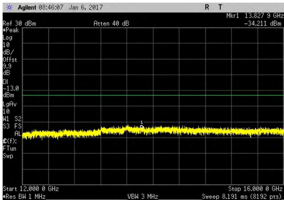
7.6_CSE_UL_1850-1915MHz_R4
