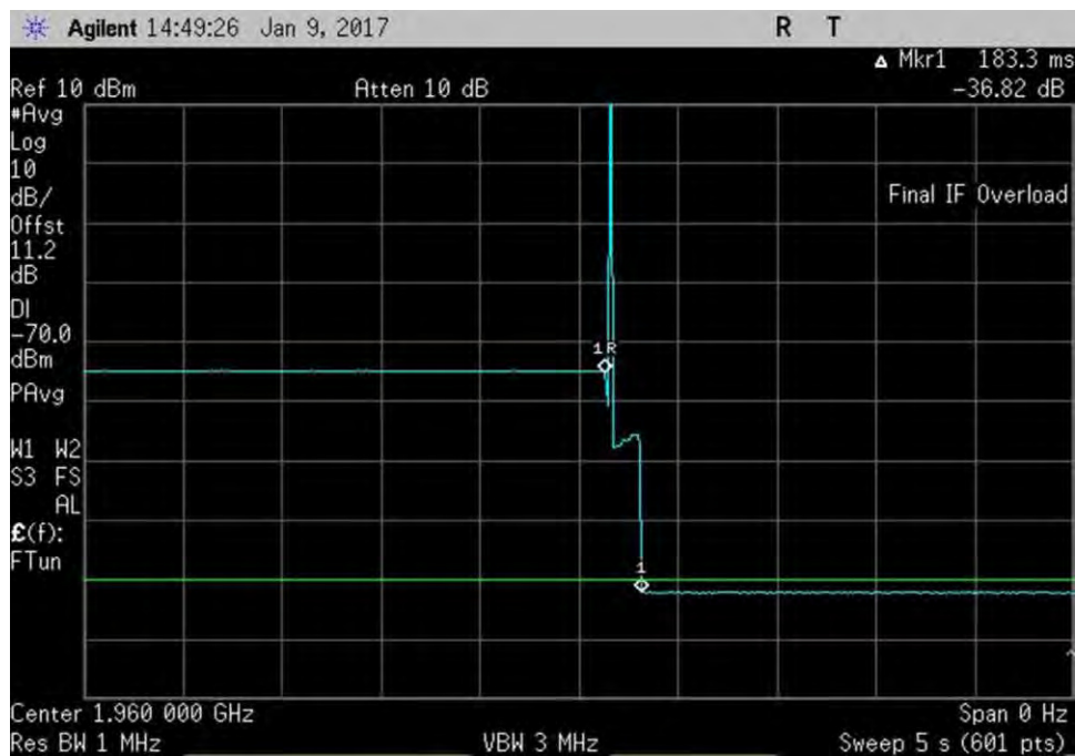
7.11.2_osc_DL_1930-1995MHz
