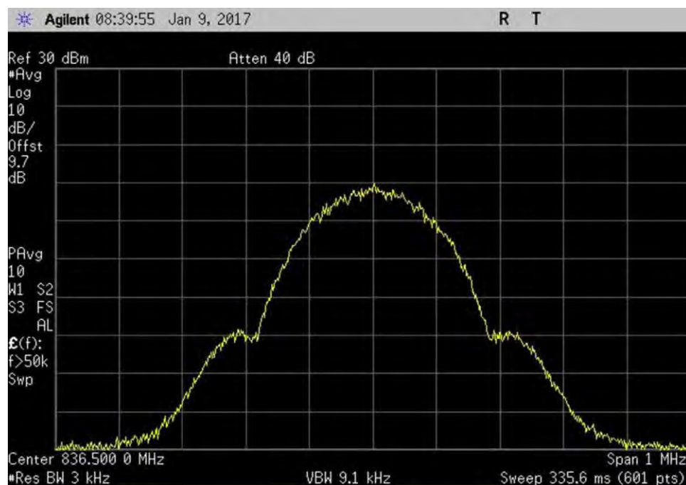
7.10_OBW_UL_824-849MHz_GSM_Out
