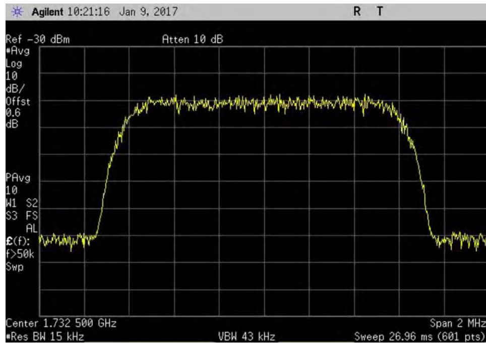
7.10_OBW_UL_1710-1755MHz_CDMA_In
