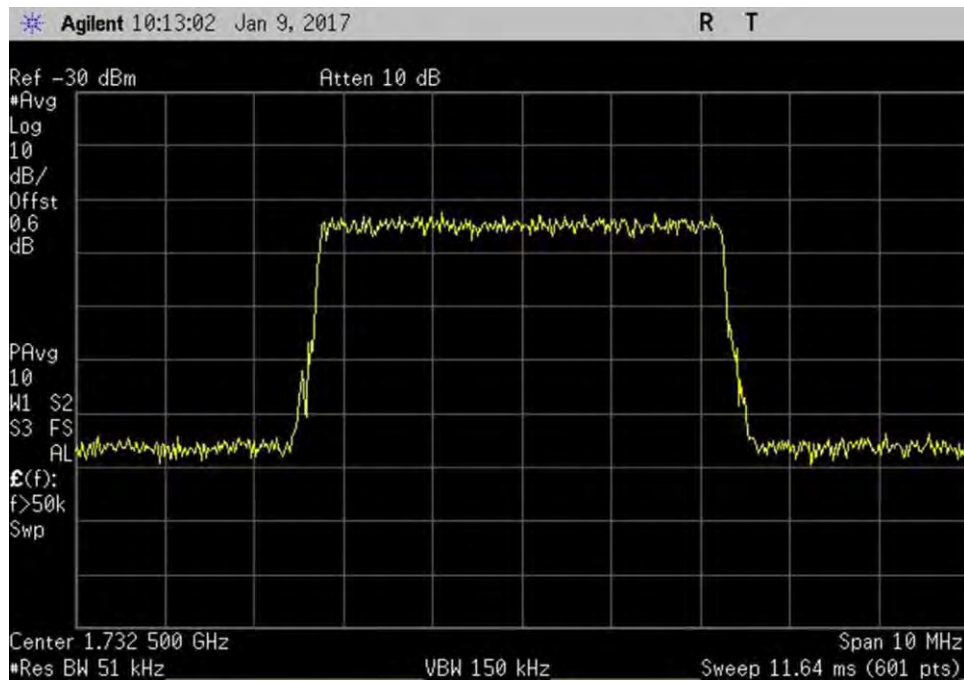
7.10_OBW_UL_1710-1755MHz_LTE_In
