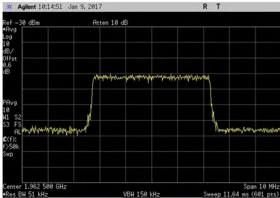
7.10_OBW_DL_1930-1995MHz_LTE_In
