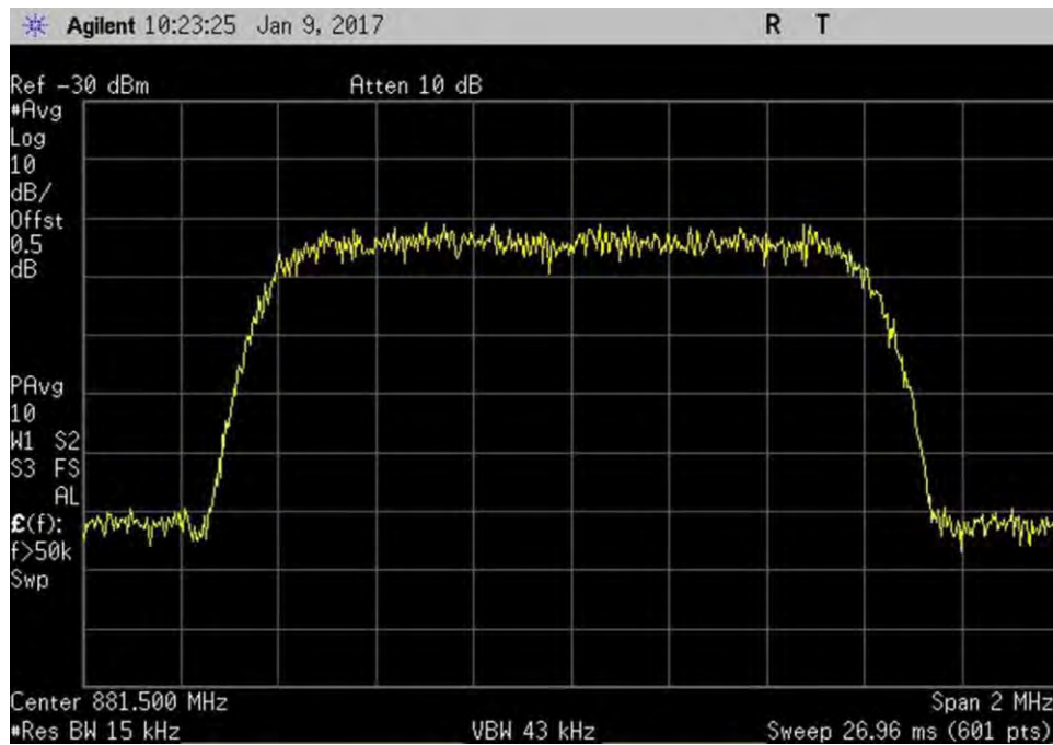
7.10_OBW_DL_869-894MHz_CDMA_In
