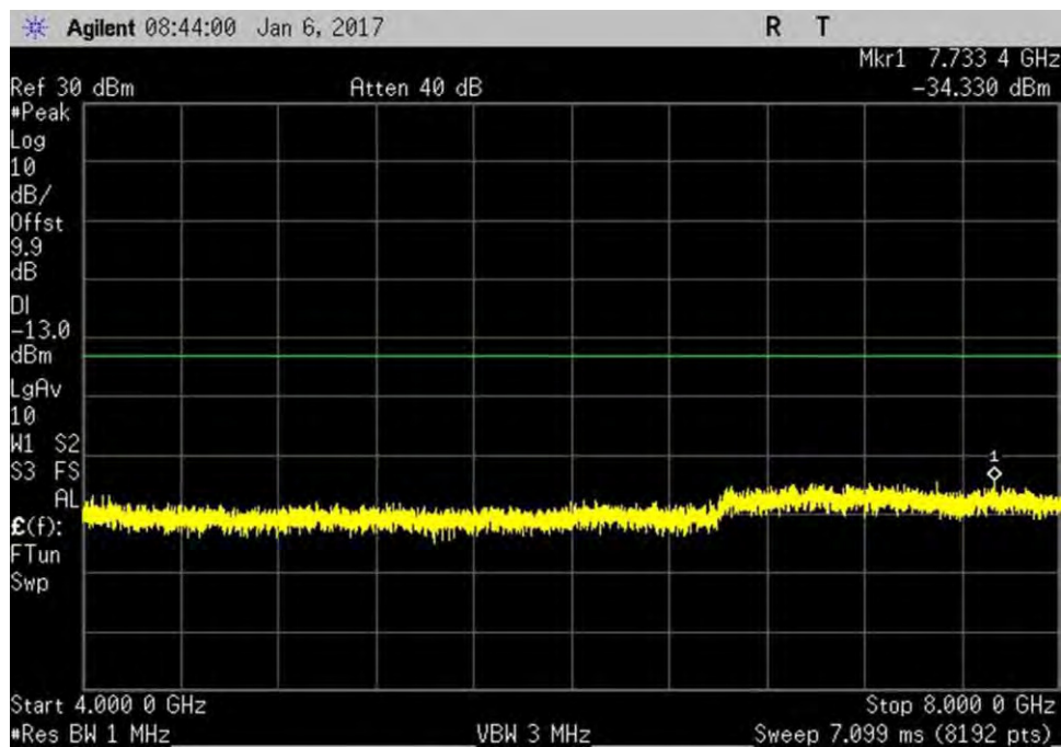
7.6_CSE_UL_1850-1915MHz_R2
