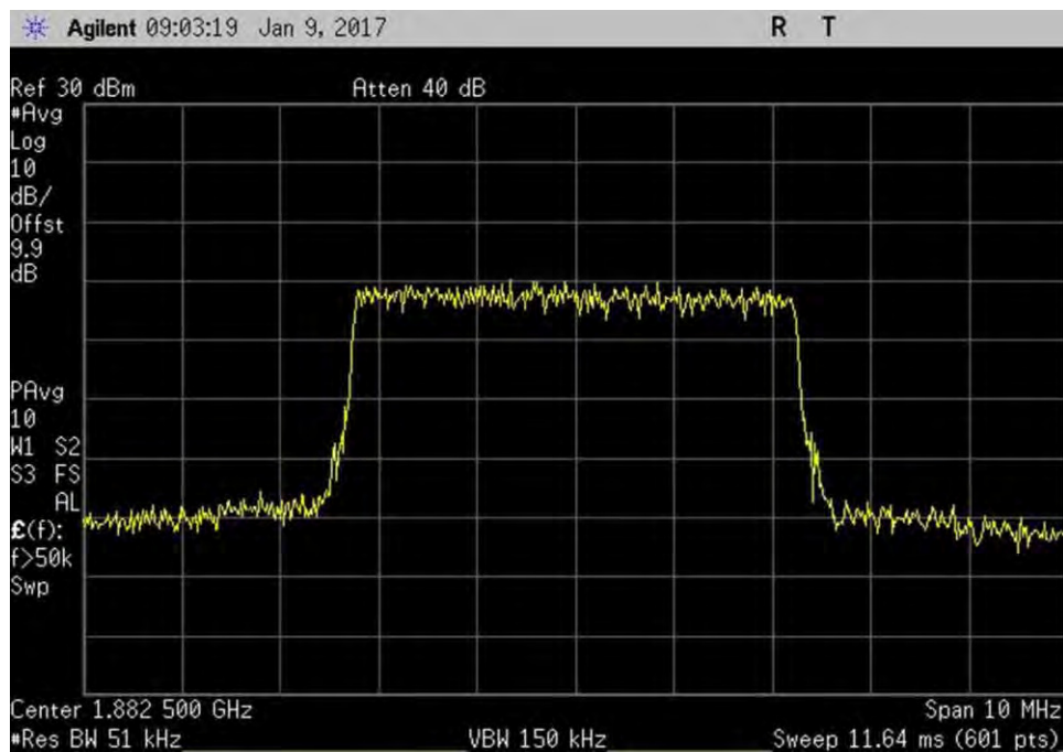
7.10_OBW_UL_1850-1915MHz_LTE_Out
