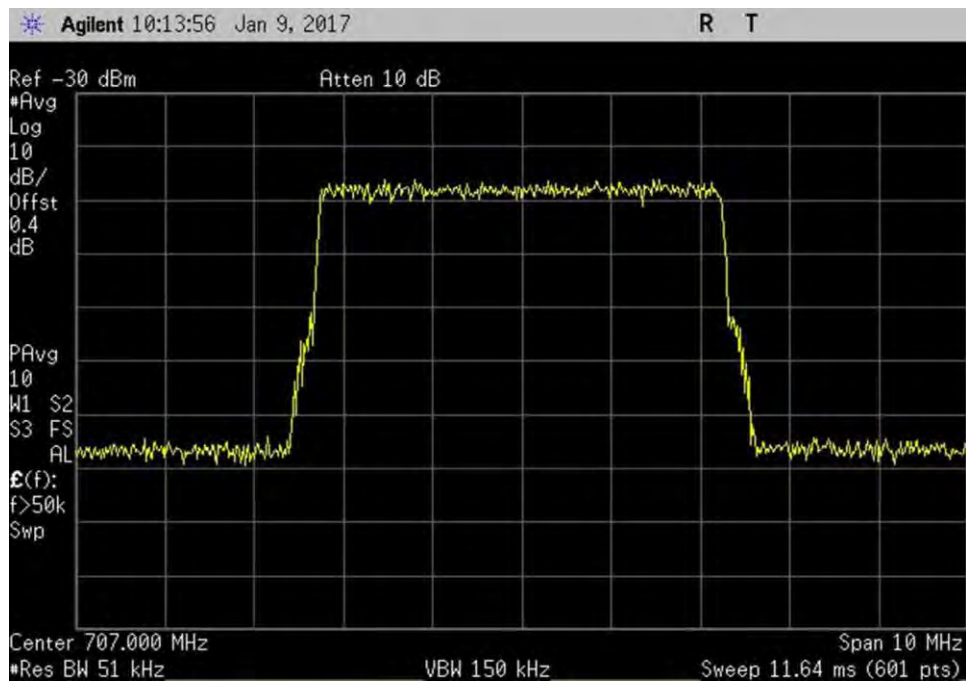
7.10_OBW_UL_698-716MHz_LTE_In
