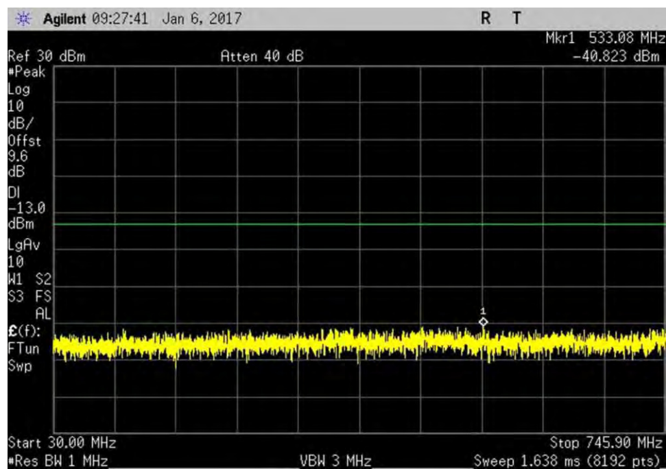
7.6_CSE_DL_746-757MHz_L
