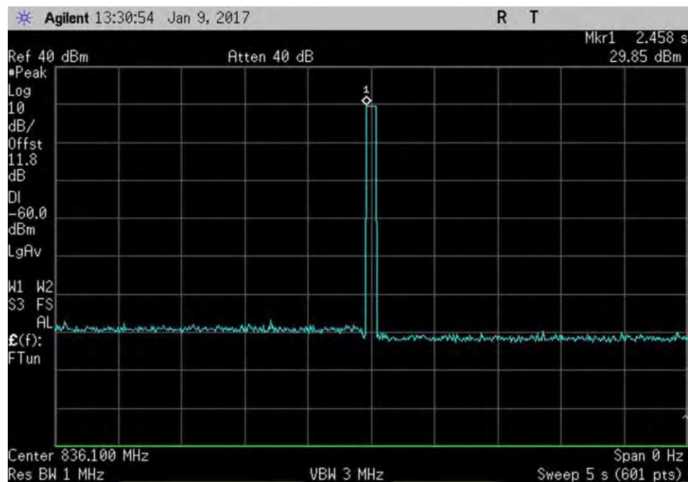
7.11.2_osc_UL_824-849MHzPk
