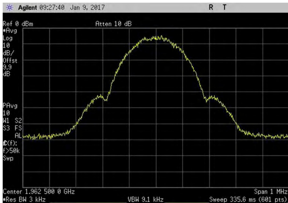
7.10_OBW_DL_1930-1995MHz_GSM_Out
