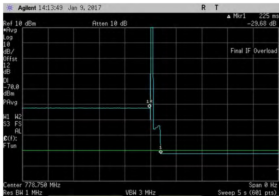
7.11.2_osc_UL_776-787MHz
