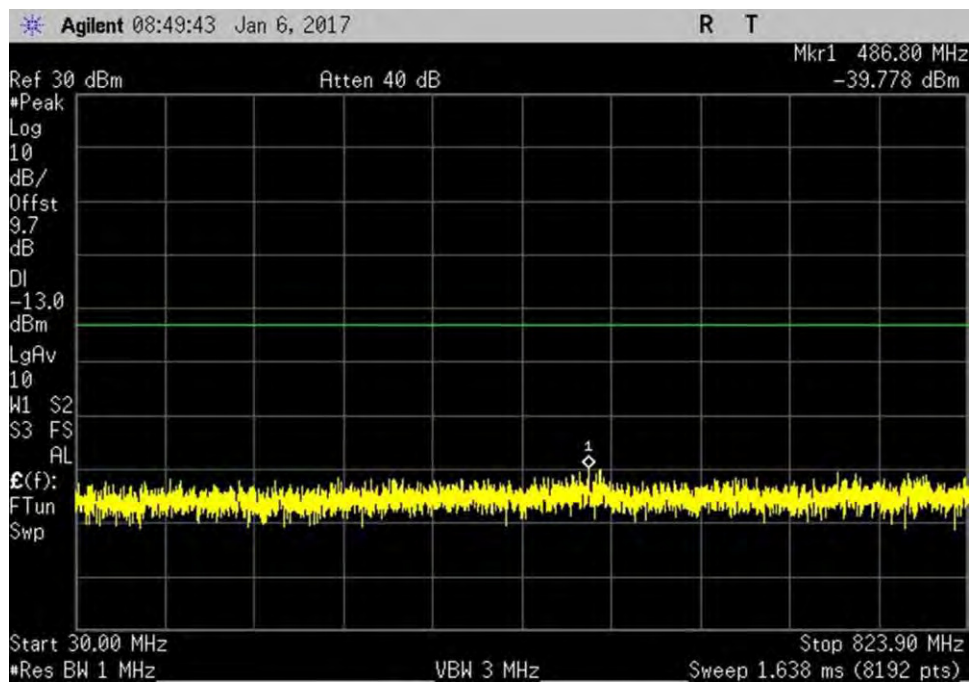
7.6_CSE_UL_824-849MHz_L
