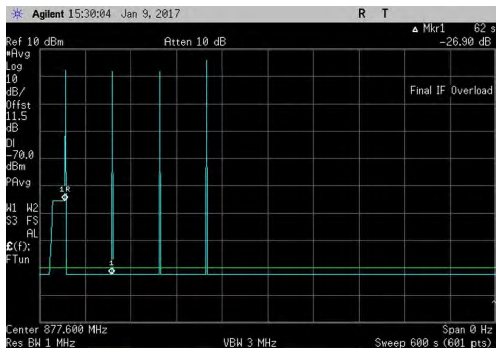
7.11.2_osc_DL_869-894MHz600sec
