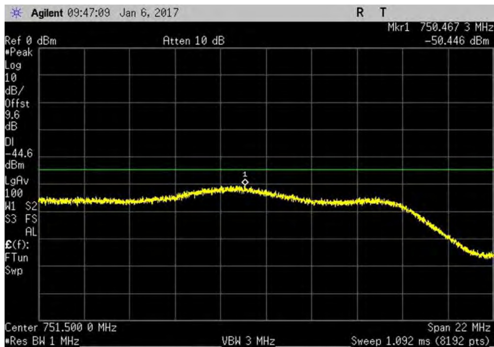
7.7.1_Noise_DL_746-757MHz
