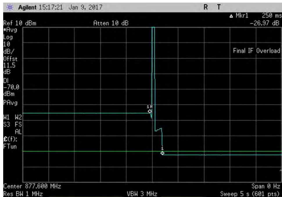
7.11.2_osc_DL_869-894MHz
