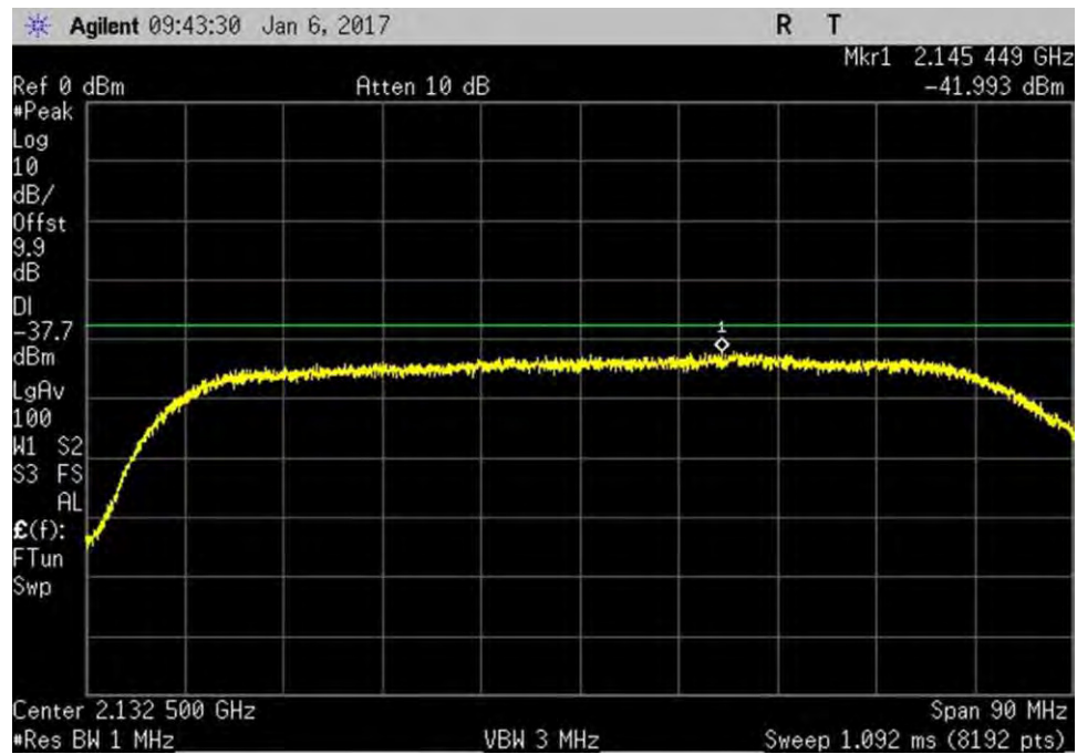
7.7.1_Noise_DL_2110-2155MHz
