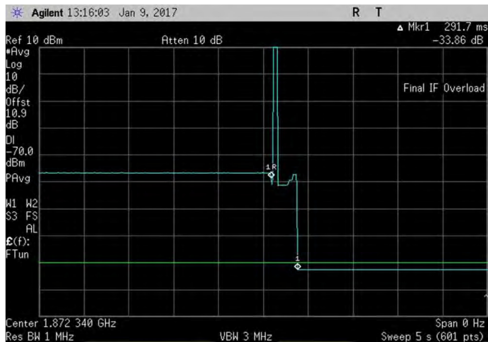
7.11.2_osc_UL_1850-1915MHz
