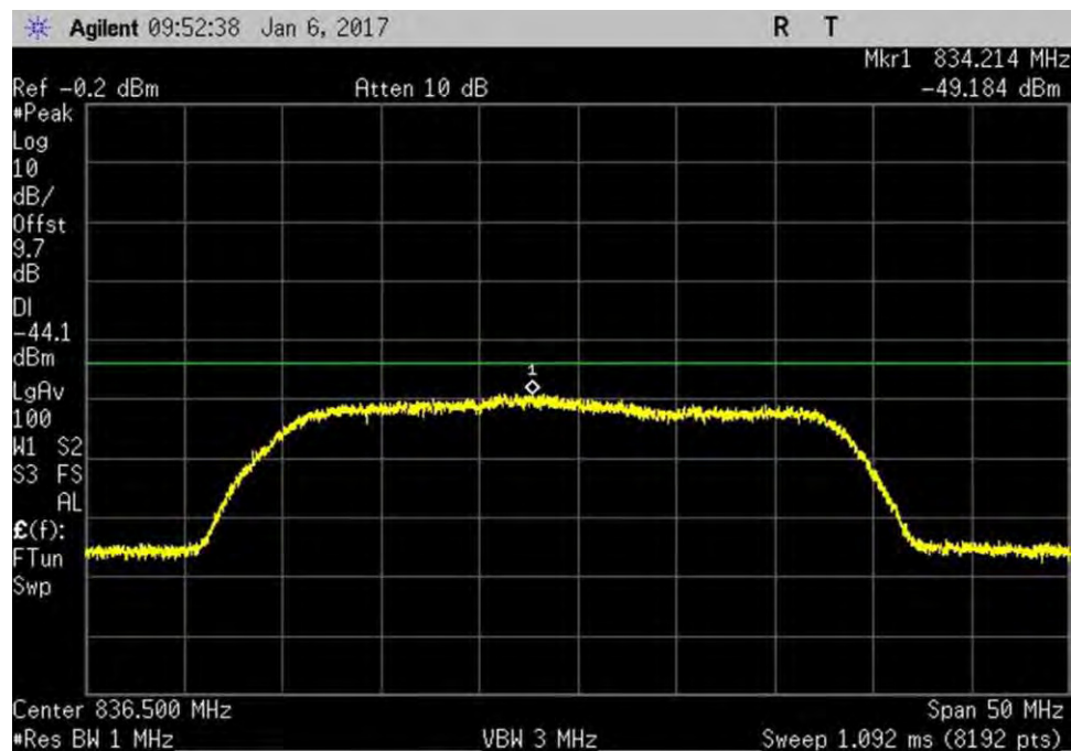
7.7.1_Noise_UL_824-849MHz
