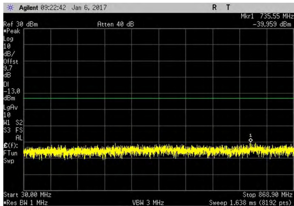
7.6_CSE_DL_869-894MHz_L
