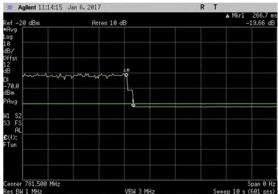
7.7.2_VarNoise_UL_776-787MHz
