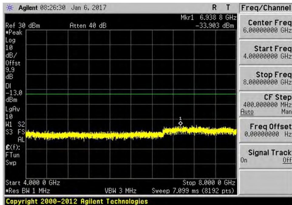
7.6_CSE_UL_1710-1755MHz_R2
