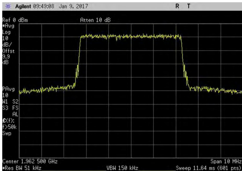
7.10_OBW_DL_1930-1995MHz_LTE_Out
