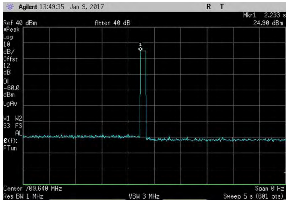
7.11.2_osc_UL_698-716MHzPk
