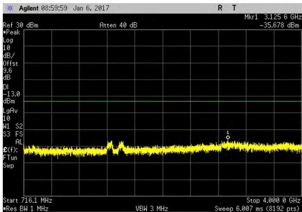
7.6_CSE_UL_698-716MHz_R1
