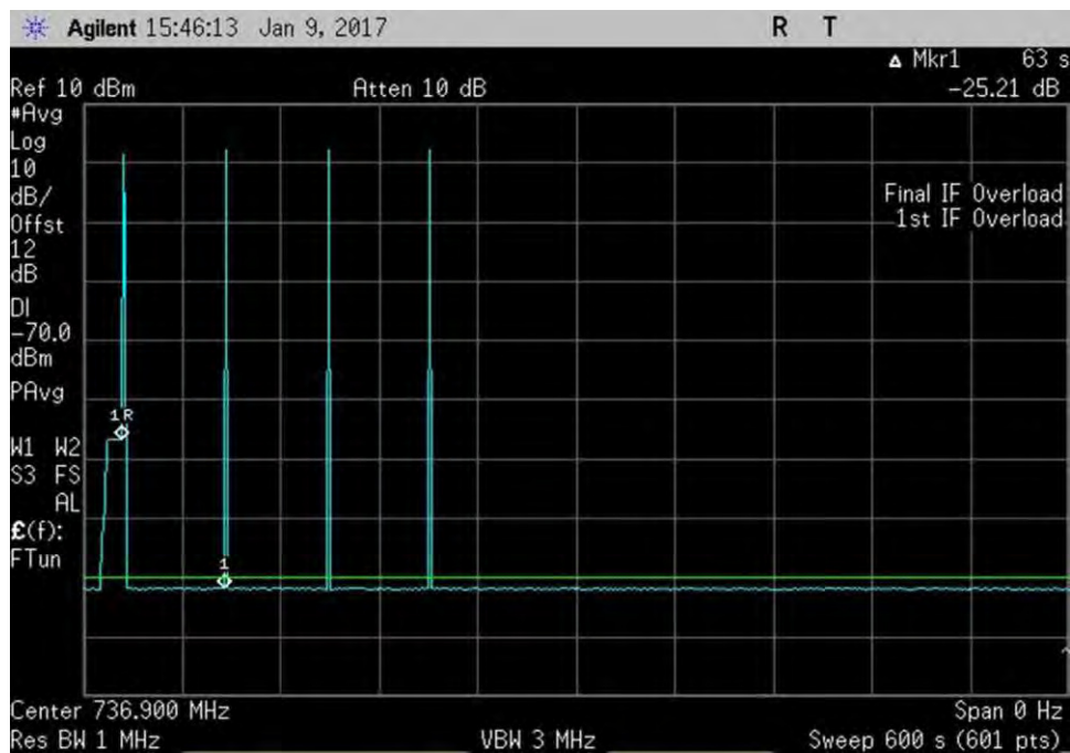
7.11.2_osc_DL_728-746MHz600sec
