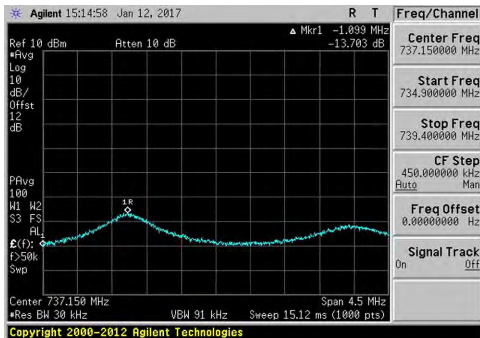
7.11.3_Osc_DL_728-746MHz+3_AWGNL
