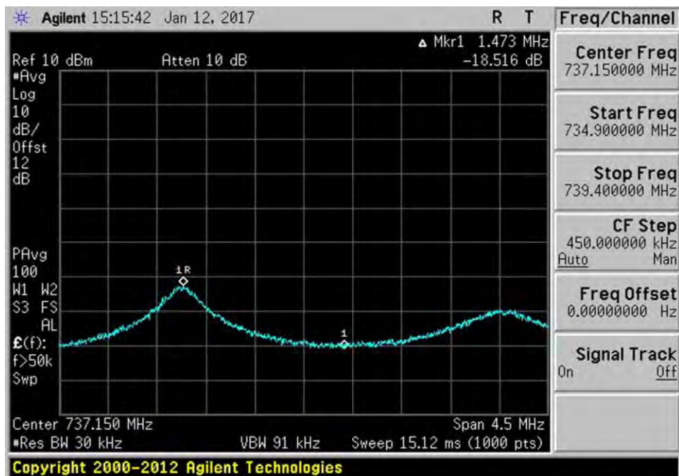
7.11.3_Osc_DL_728-746MHz+1_AWGNL
