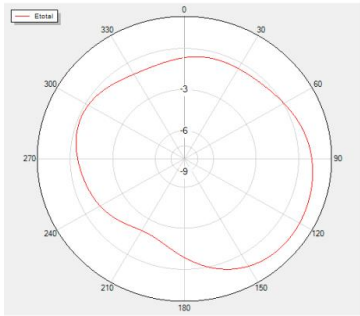
Theta=90 Freq=2500MHz
