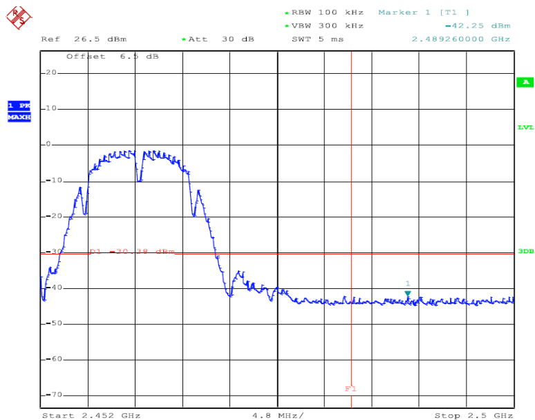
802.11b High Band Edge Plot
