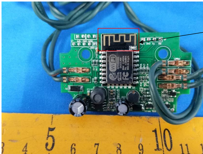
Antenna
