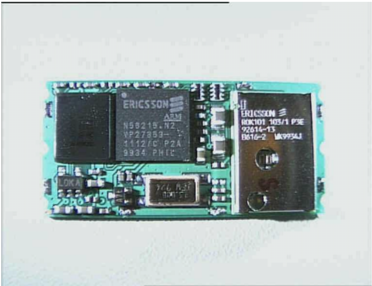
PCB top
