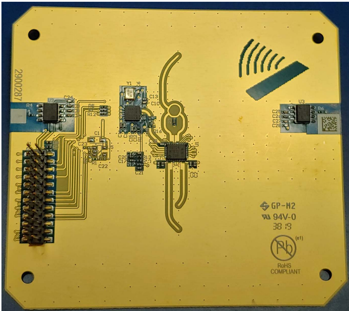
Antenna PCA Back
