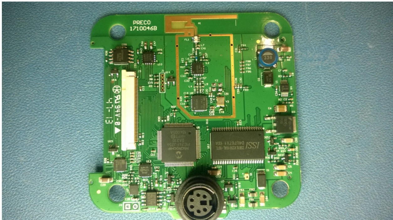
WD7102 PCB Top
