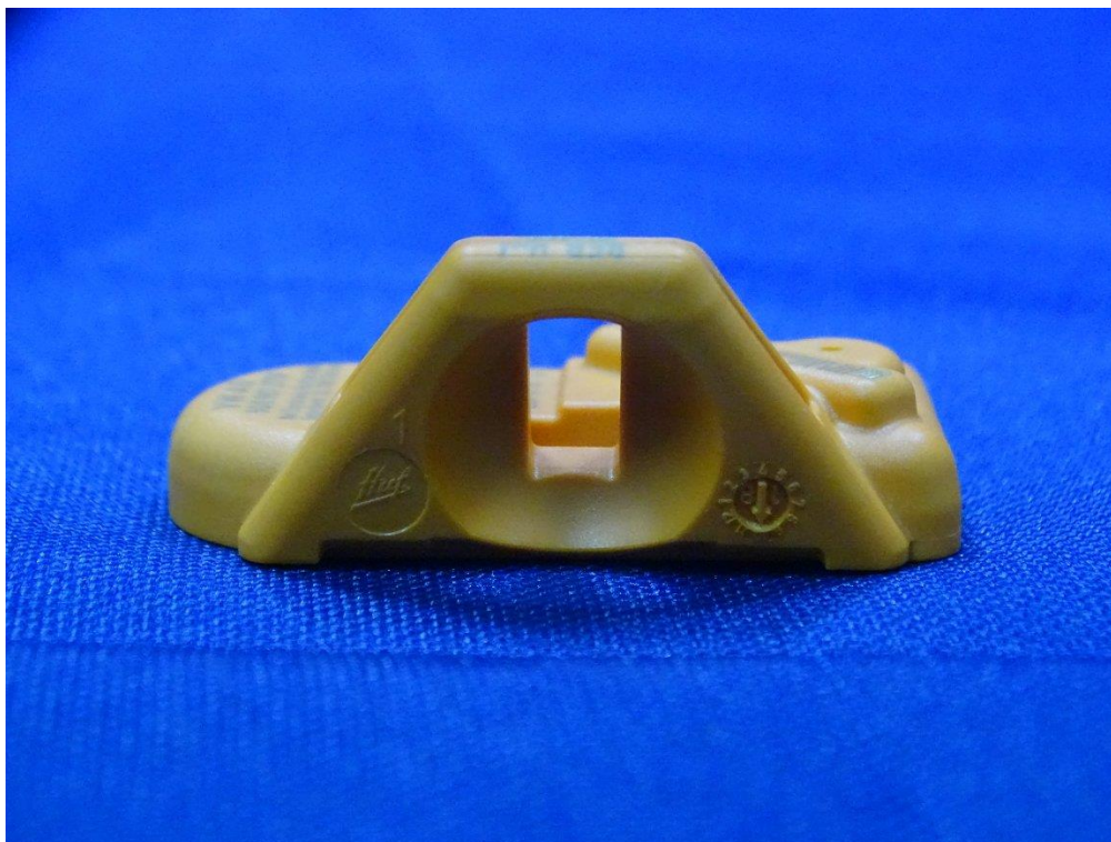
(5) EUT Photo
