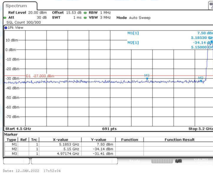
11A_Ant1_Low_5180
