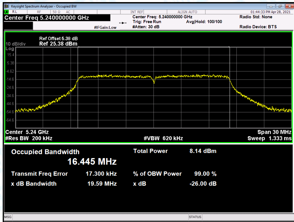
OBW NVNT a 5240MHz Ant.B
