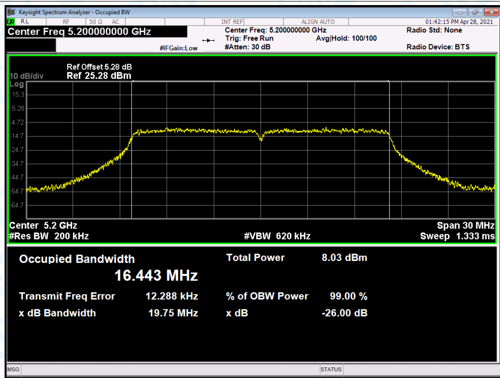
OBW NVNT a 5200MHz Ant.B
