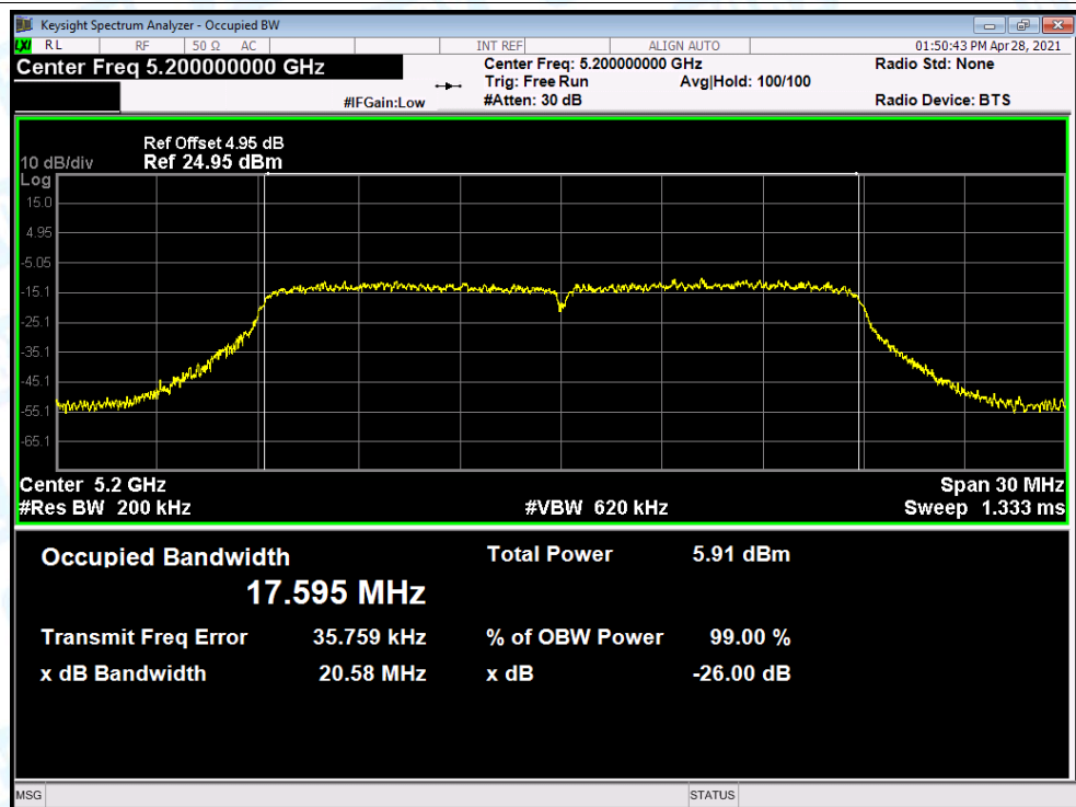
OBW NVNT n(HT20) 5200MHz Ant.B
