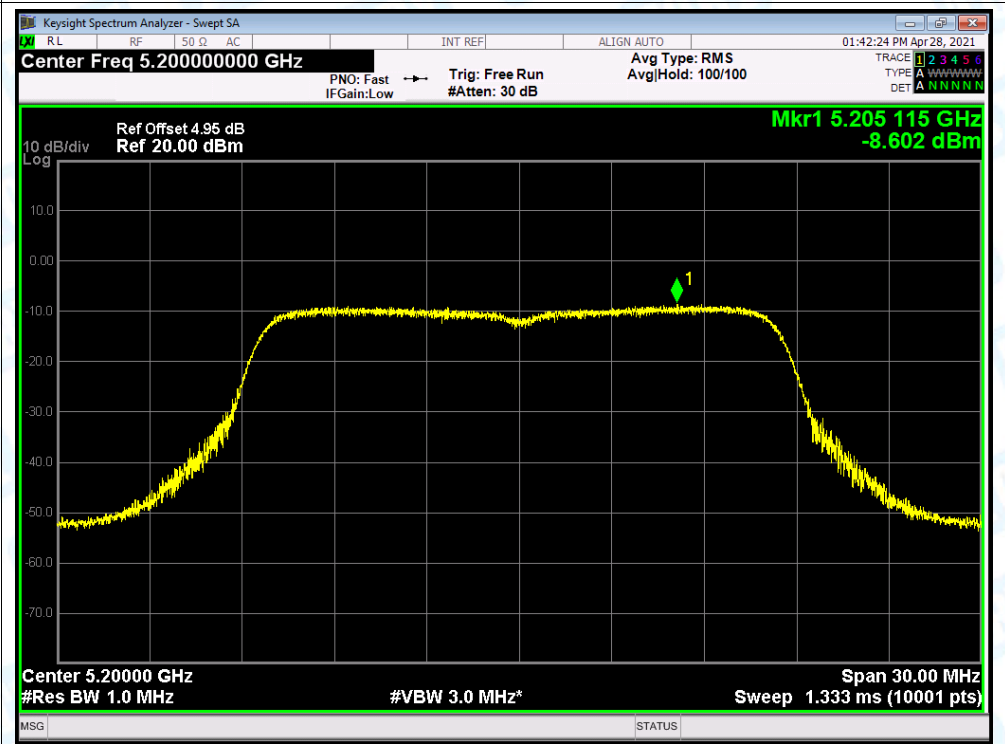
PSD NVNT a 5200MHz Ant.B
