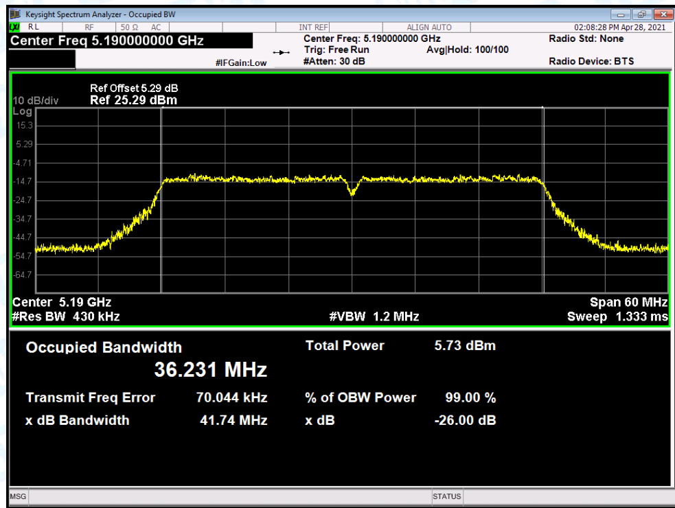
OBW NVNT n(HT40) 5190MHz Ant.B
