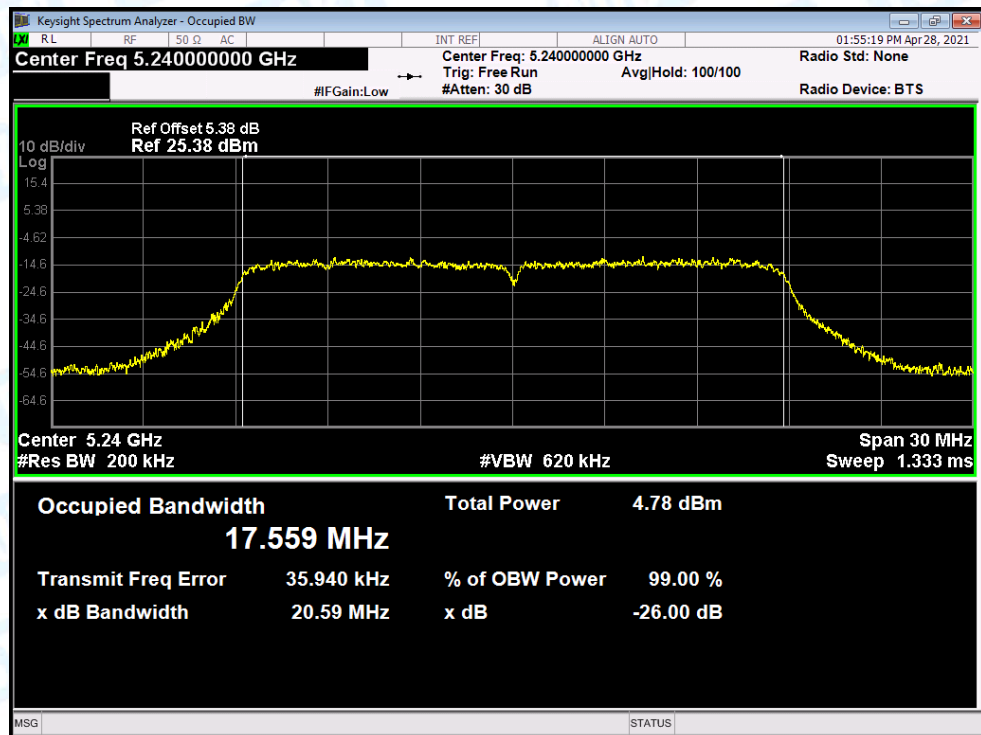
OBW NVNT n(HT20) 5240MHz Ant.B
