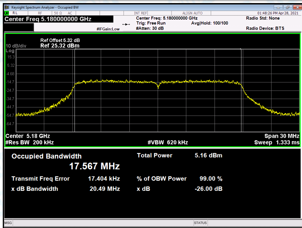
OBW NVNT n(HT20) 5180MHz Ant.B
