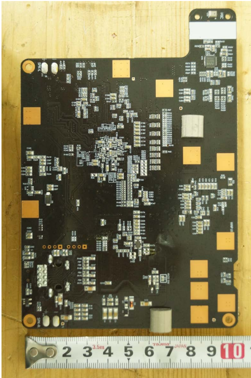
<Main PCB>
