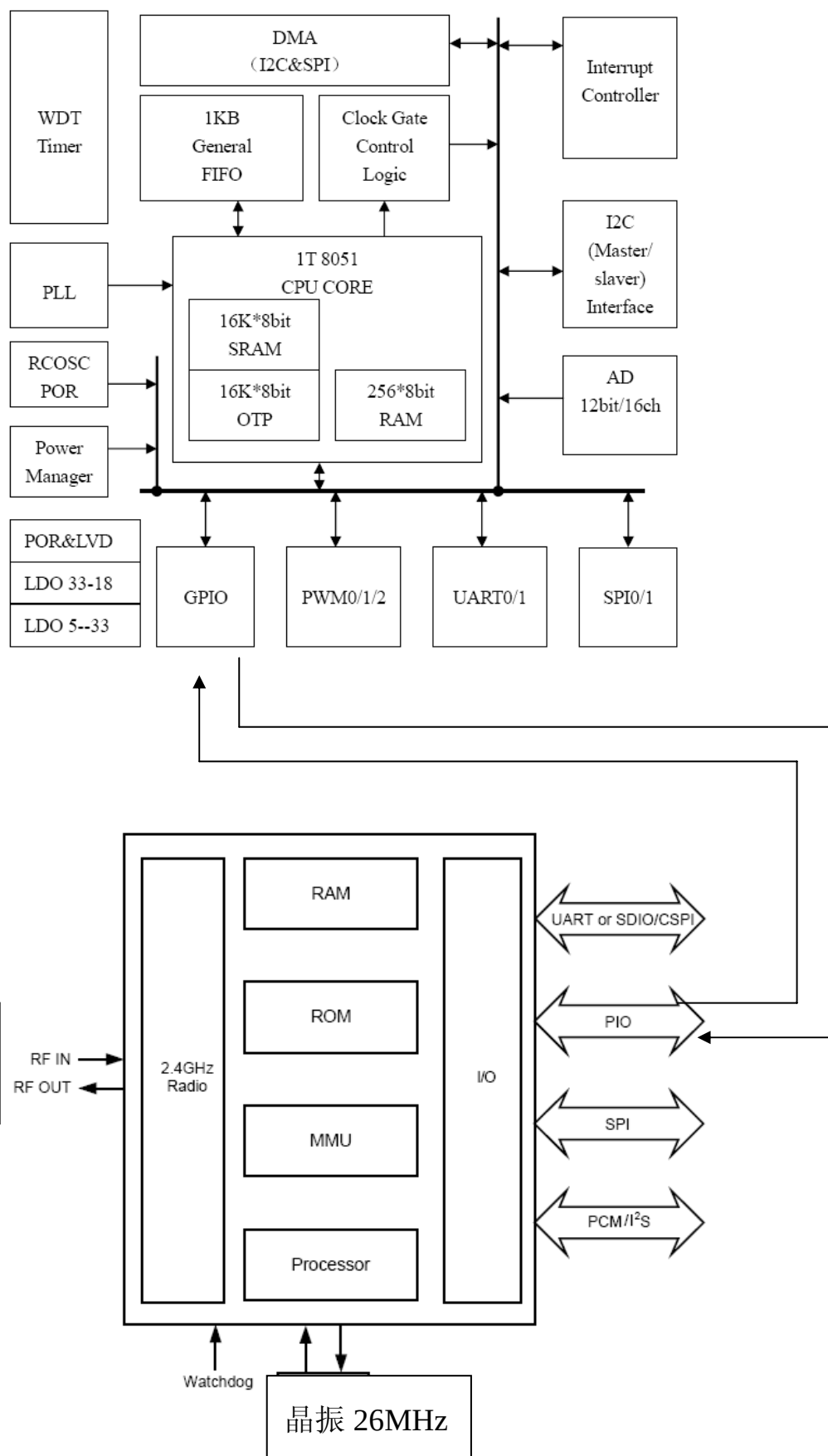
MARB0201 方框图
