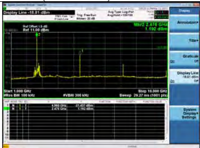
2480MHz(2.4GHz – 2.5GHz)
