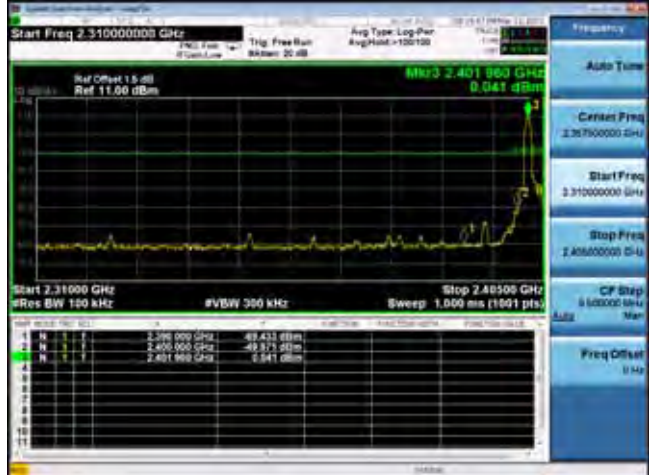
2402MHz(2.3GHz – 2.4GHz)
