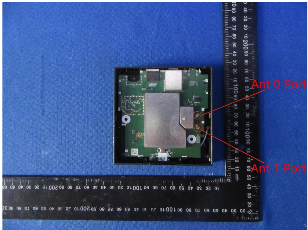
(3) EUT Photo
