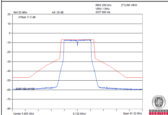
802.11be (EHT20) / Chain 1 : CH 1
