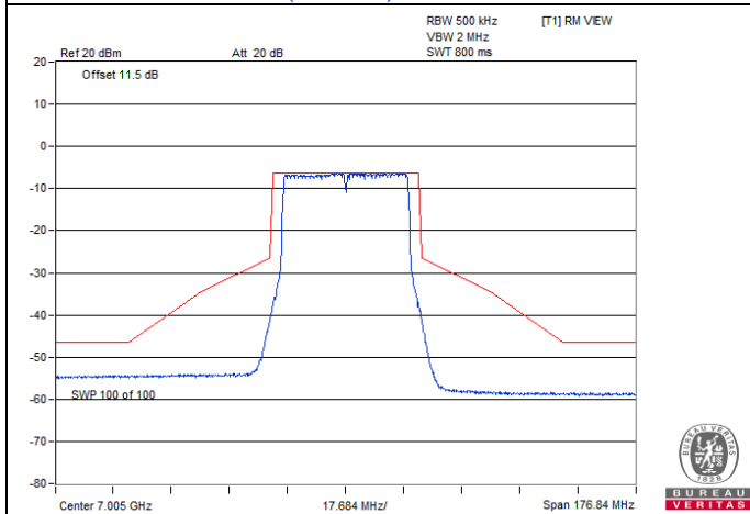
802.11be (EHT40) / Chain 2 : CH 211
