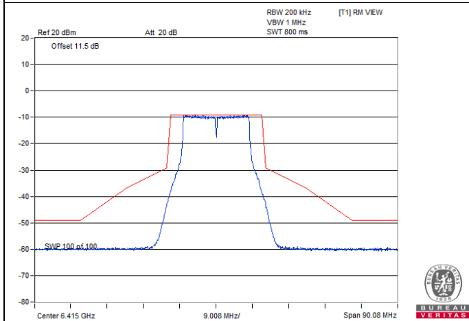
802.11a / Chain 3 : CH 93
