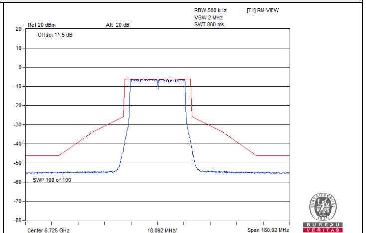
802.11be (EHT40) / Chain 2 : CH 155
