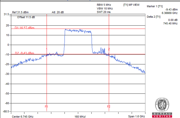
802.11be (EHT320) / Chain 1 : CH 159
