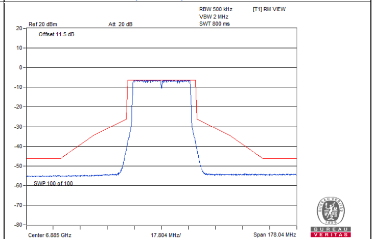
802.11be (EHT40) / Chain 2 : CH 187
