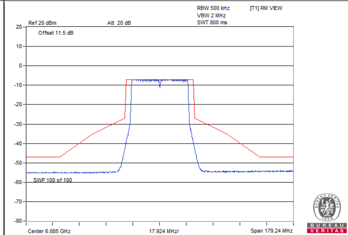
802.11be (EHT40) / Chain 3 : CH 187
