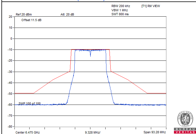
802.11be (EHT20) / Chain 1 : CH 105
