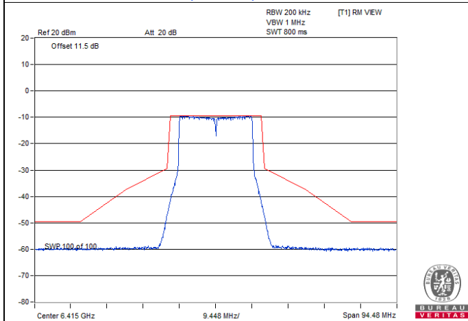
802.11be (EHT20) / Chain 1 : CH 93
