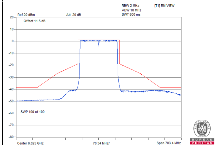
802.11be (EHT160) / Chain 3 : CH 15
