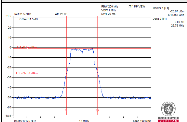
802.11a / Chain 3 : CH 45
