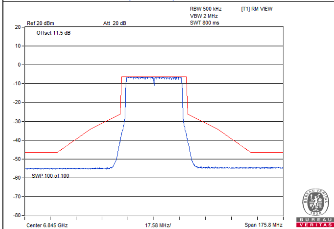
802.11be (EHT40) / Chain 2 : CH 179
