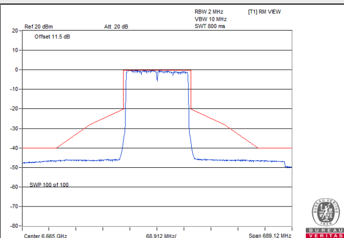
802.11be (EHT160) / Chain 3 : CH 143
