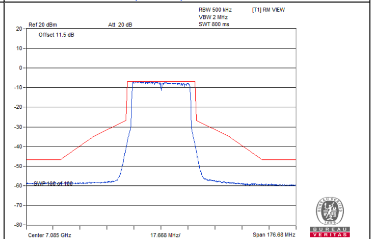
802.11be (EHT40) / Chain 2 : CH 227
