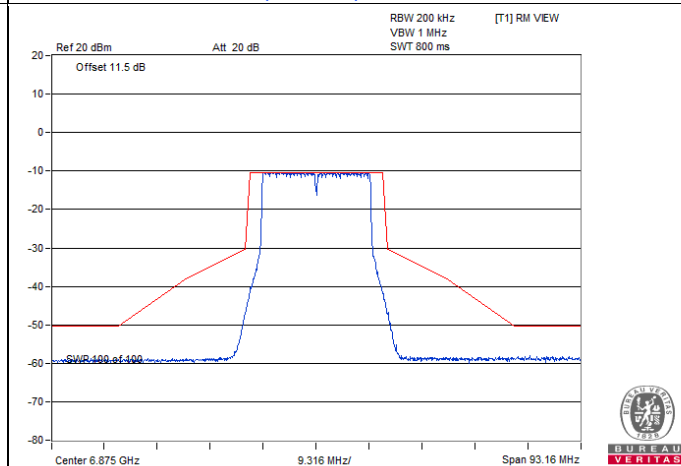
802.11be (EHT20) / Chain 2 : CH 185
