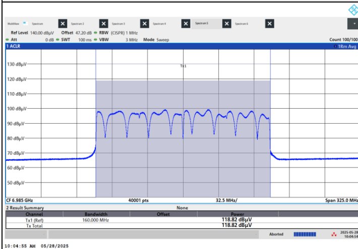
802.11be (EHT160) CDD : CH 207
