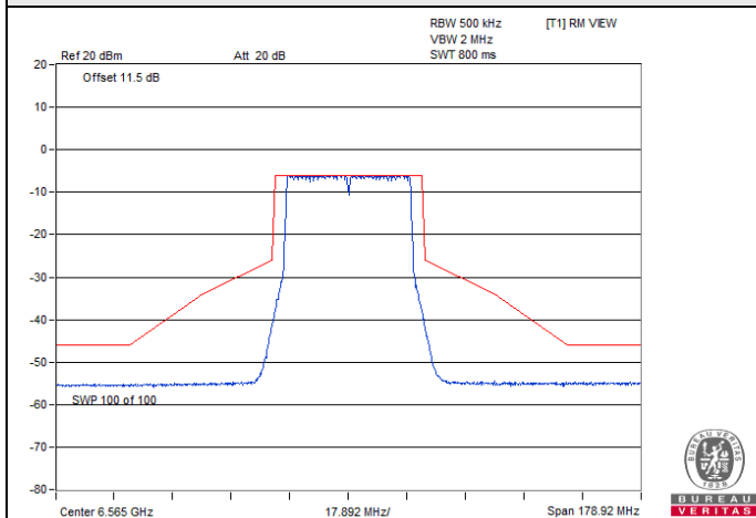
802.11be (EHT40) / Chain 2 : CH 123
