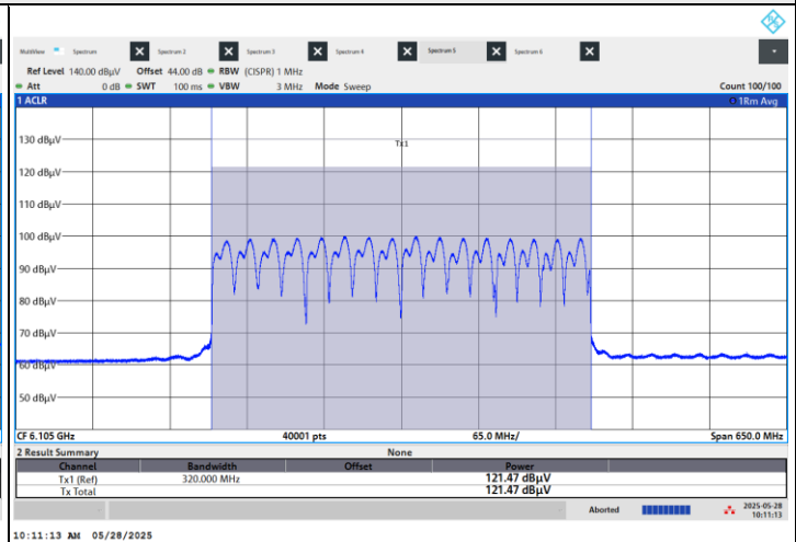
802.11be (EHT320) CDD : CH 31
