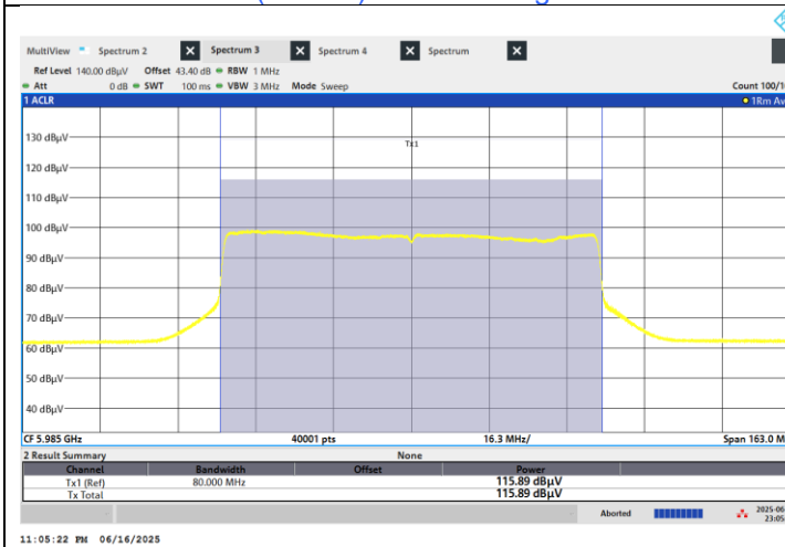
802.11be (EHT80) Beamforming : CH 7
