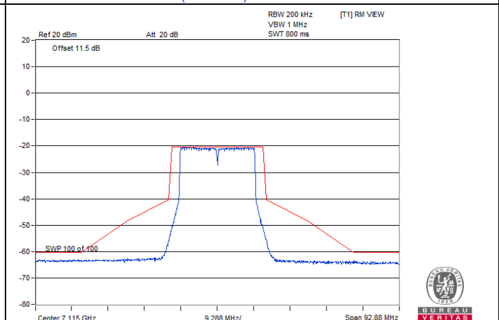
802.11be (EHT20) / Chain 3 : CH 233
