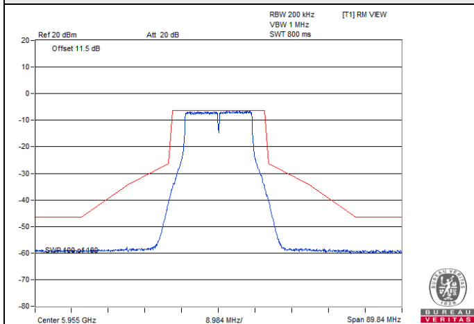
802.11a / Chain 3 : CH 1
