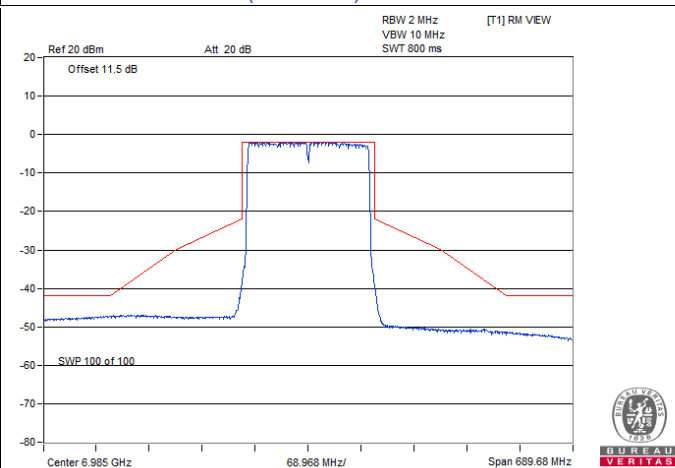
802.11be (EHT160) / Chain 3 : CH 207
