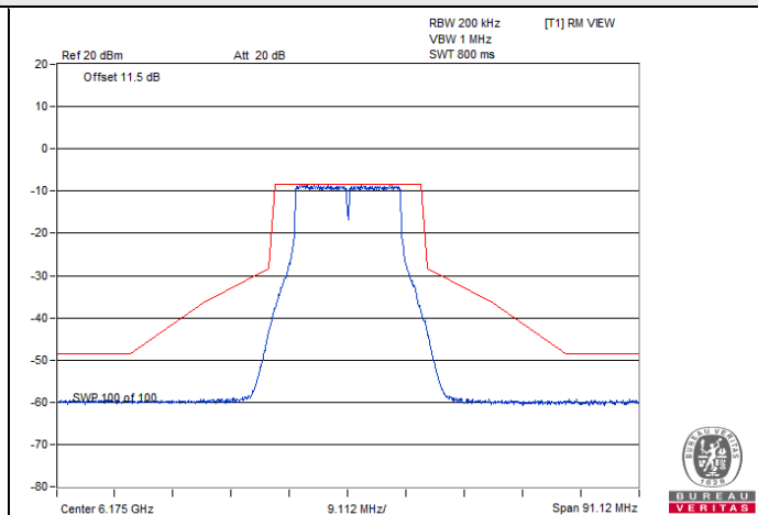
802.11a / Chain 3 : CH 45
