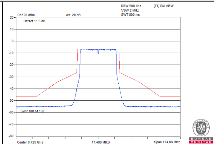
802.11be (EHT40) / Chain 3 : CH 155
