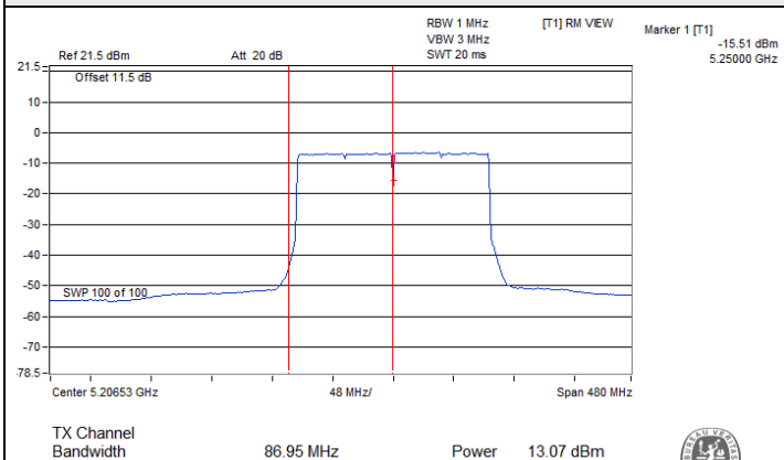
802.11be (EHT160) CDD / Chain 2 : CH 50 (U-NII-1)
