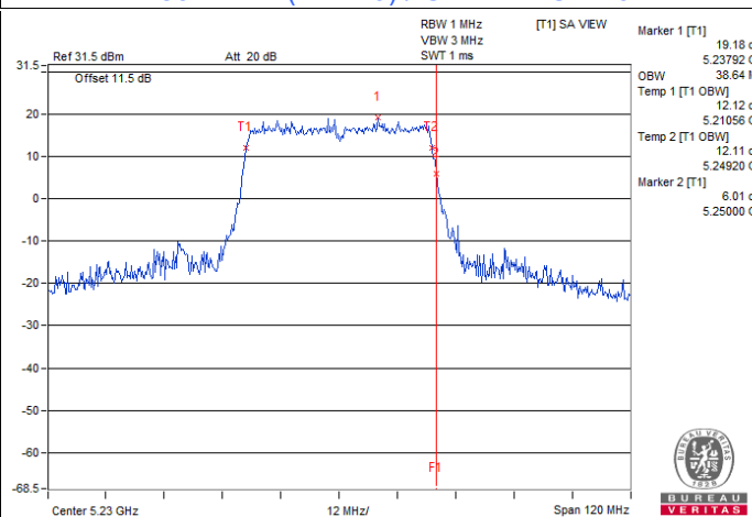
802.11be (EHT40) / Chain 3 : CH 46
