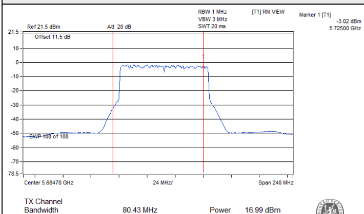
802.11be (EHT80) CDD / Chain 3 : CH 138 (U-NII-2C)
