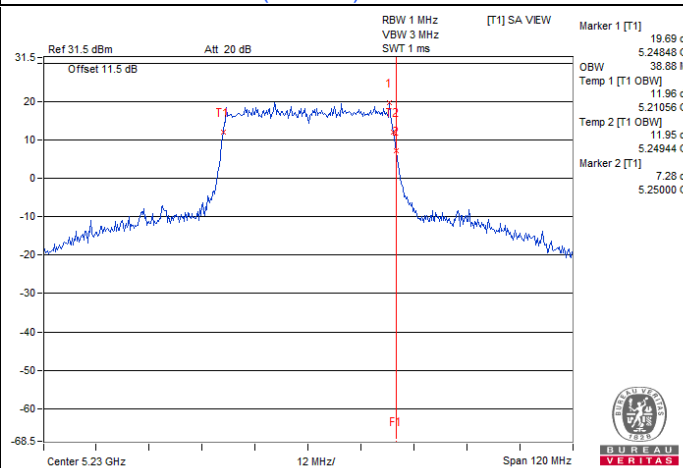
802.11be (EHT40) / Chain 1 : CH 46
