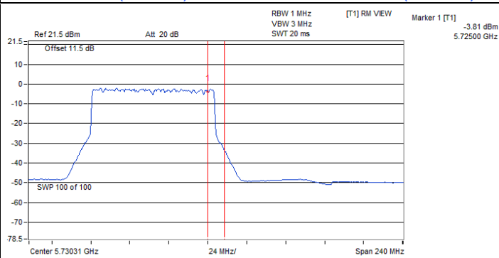
802.11be (EHT80) CDD / Chain 1 : CH 138 (U-NII-3)
