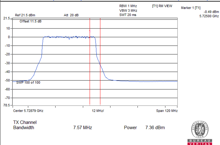
802.11be (EHT40) CDD / Chain 3 : CH 142 (U-NII-3)
