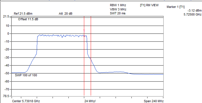
802.11be (EHT80) CDD / Chain 0 : CH 138 (U-NII-3)
