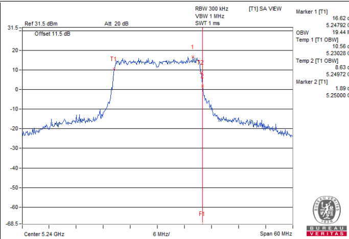
802.11be (EHT20) / Chain 3 : CH 48
