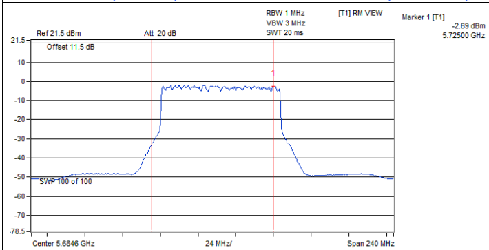
802.11be (EHT80) CDD / Chain 1 : CH 138 (U-NII-2C)
