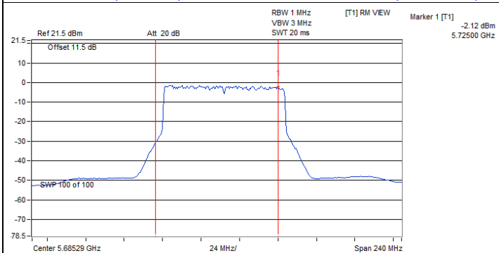
802.11be (EHT80) CDD / Chain 0 : CH 138 (U-NII-2C)
