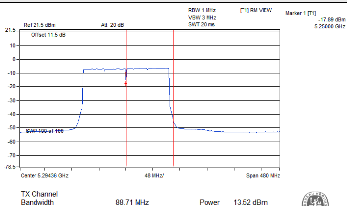
802.11be (EHT160) CDD / Chain 2 : CH 50 (U-NII-2A)
