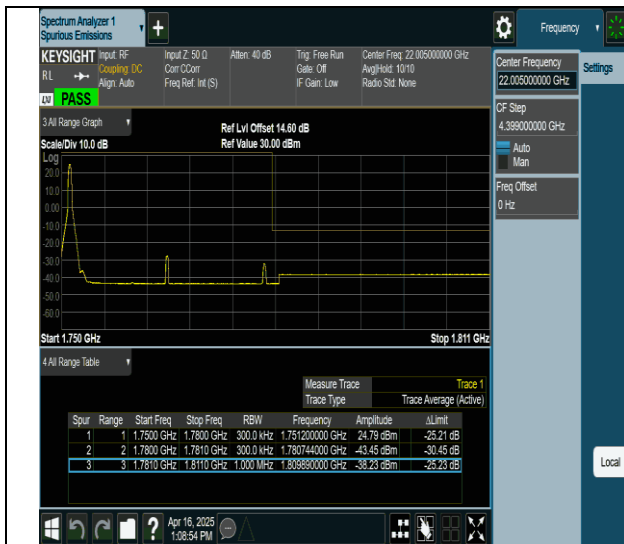
66-66-20MHz-10MHz-QPSK@QPSK-QPSK@QPSK-132473- 132617-1RB#0@0RB#0-0RB#0@0RB#0-PASS
