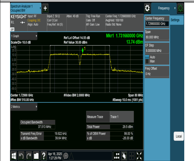
66-66-20MHz-20MHz-16QAM-16QAM-132072-132270-100RB#0-100RB#0-PASS
