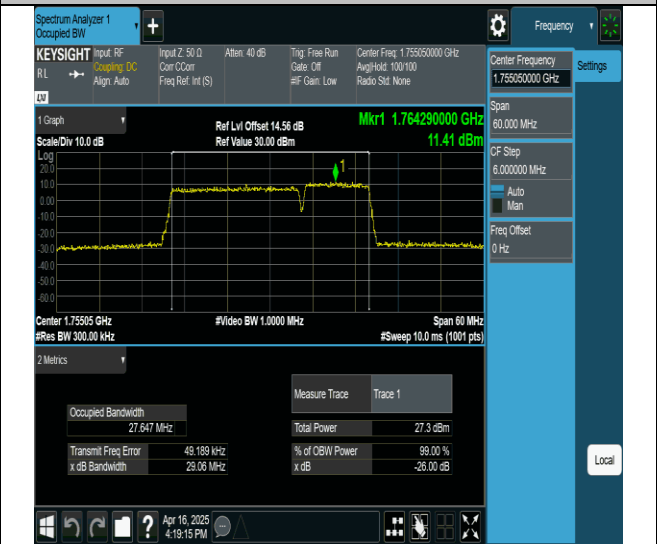
66-66-20MHz-10MHz-256QAM-256QAM-132373-132517-100RB#0-50RB#0-PASS
