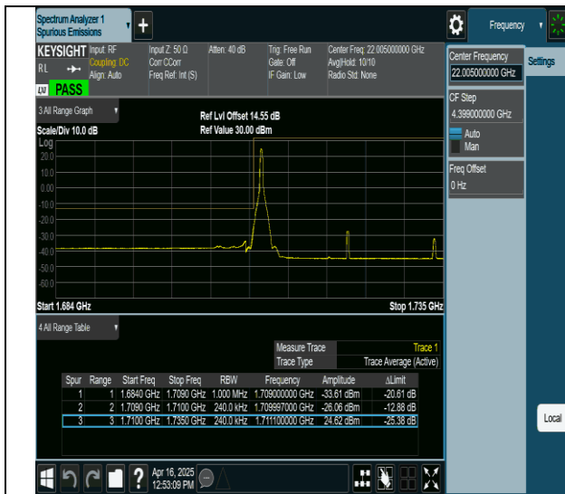
66-66-20MHz-5MHz-QPSK@QPSK-QPSK@QPSK-132072-132189-1RB#0@0RB#0-0RB#0@0RB#0-PASS
