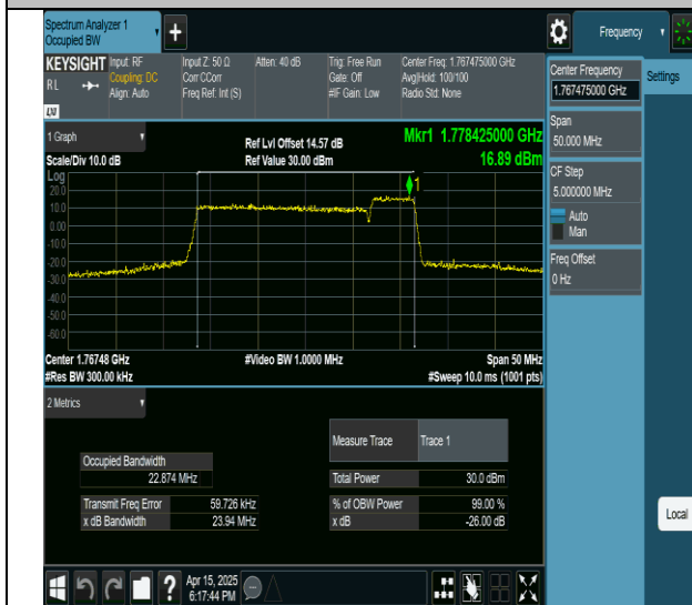
66-66-20MHz-5MHz-QPSK-QPSK-132522-132639-100RB#0-25RB#0-PASS
