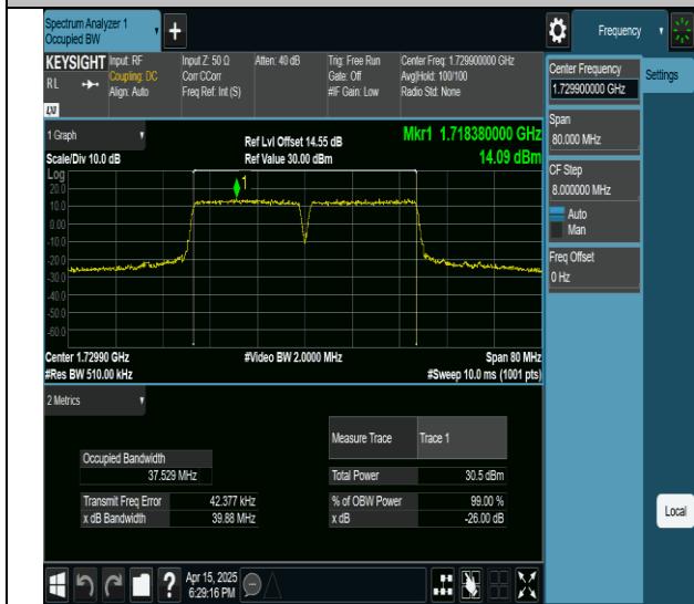
66-66-20MHz-20MHz-QPSK-QPSK-132072-132270-100RB#0-100RB#0-PASS
