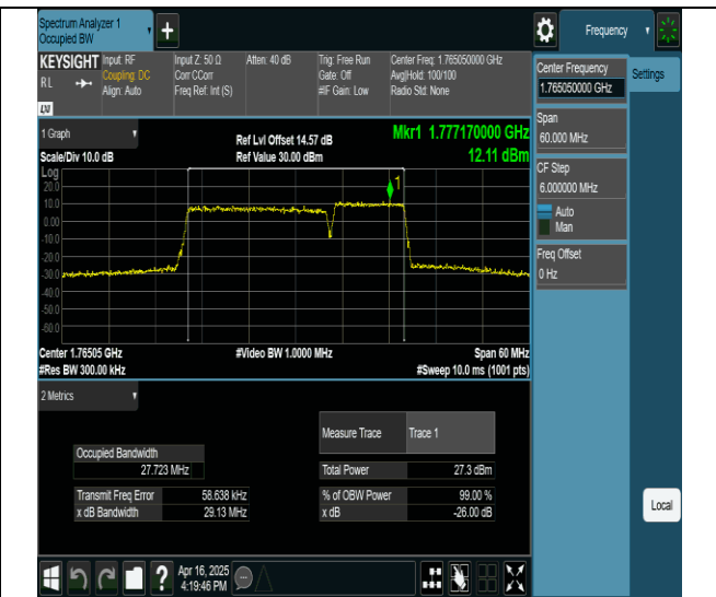
66-66-20MHz-10MHz-256QAM-256QAM-132473-132617-100RB#0-50RB#0-PASS
