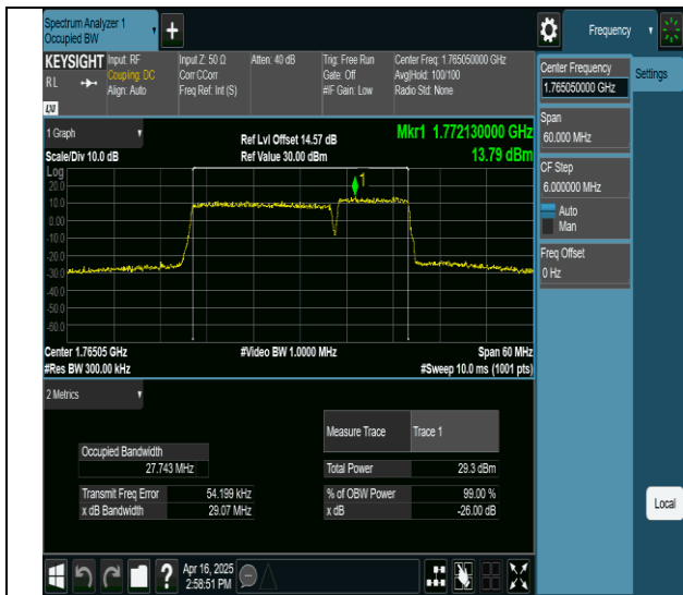
66-66-20MHz-10MHz-64QAM-64QAM-132473-132617-100RB#0-50RB#0-PASS
