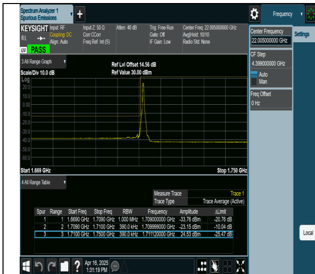
66-66-20MHz-20MHz-QPSK@QPSK-QPSK@QPSK-132072- 132270-1RB#0@0RB#0-0RB#0@0RB#0-PASS
