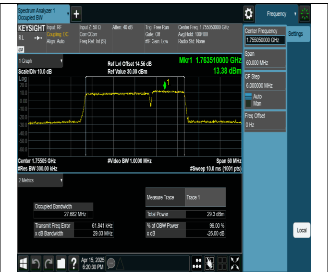
66-66-20MHz-10MHz-16QAM-16QAM-132373-132517-100RB#0-50RB#0-PASS
