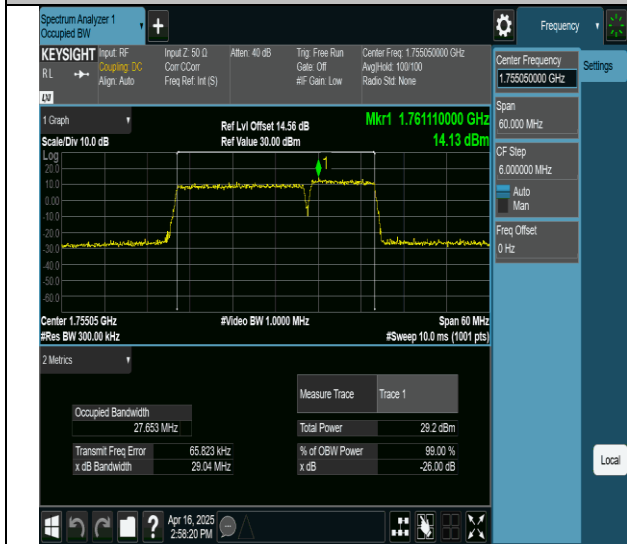
66-66-20MHz-10MHz-64QAM-64QAM-132373-132517-100RB#0-50RB#0-PASS
