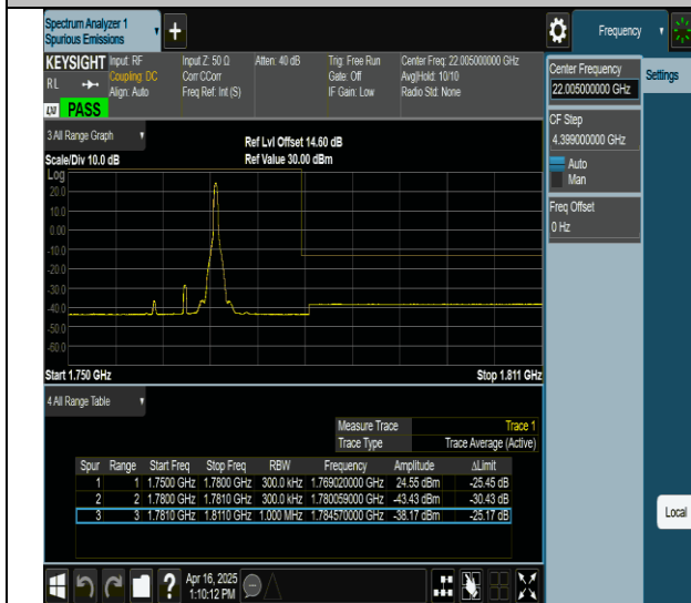
66-66-20MHz-10MHz-QPSK@QPSK-QPSK@QPSK-132473- 132617-1RB#99@0RB#0-0RB#0@0RB#0-PASS
