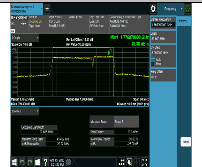
66-66-20MHz-10MHz-16QAM-16QAM-132473-132617-100RB#0-50RB#0-PASS
