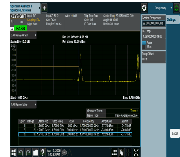
66-66-20MHz-20MHz-QPSK@QPSK-QPSK@QPSK-132072- 132270-1RB#0@0RB#0-1RB#99@0RB#0-PASS
