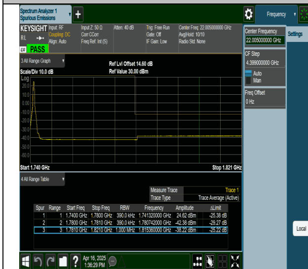
66-66-20MHz-20MHz-QPSK@QPSK-QPSK@QPSK-132374- 132572-1RB#0@0RB#0-0RB#0@0RB#0-PASS
