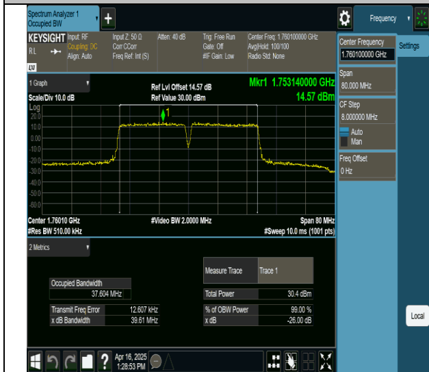
66-66-20MHz-20MHz-QPSK-QPSK-132374-132572-100RB#0-100RB#0-PASS
