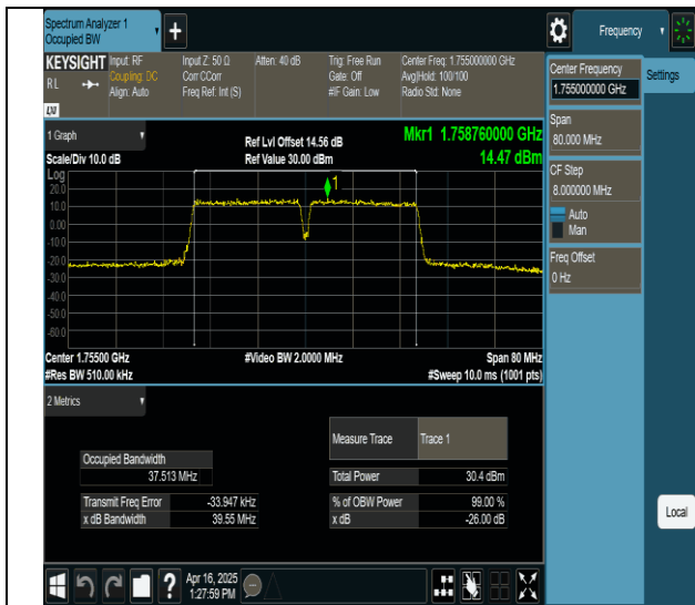
66-66-20MHz-20MHz-QPSK-QPSK-132323-132521-100RB#0-100RB#0-PASS
