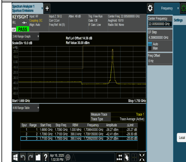
66-66-20MHz-20MHz-QPSK@QPSK-QPSK@QPSK-132072- 132270-1RB#99@0RB#0-0RB#0@0RB#0-PASS
