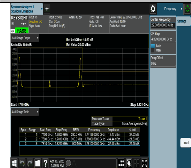
66-66-20MHz-20MHz-QPSK@QPSK-QPSK@QPSK-132374- 132572-1RB#0@0RB#0-1RB#99@0RB#0-PASS
