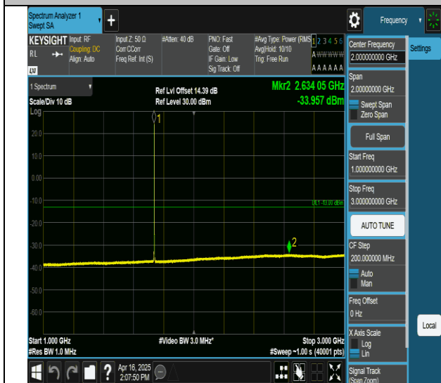
66-66-20MHz-20MHz-QPSK-QPSK-132323-132521-1RB#0- ORB#0-1000~3000MHz-PASS
