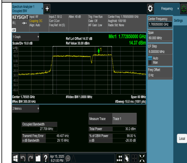
66-66-20MHz-10MHz-QPSK-QPSK-132473-132617-100RB#0-50RB#0-PASS
