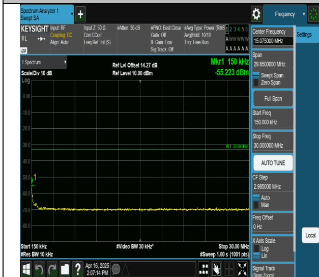
66-66-20MHz-20MHz-QPSK-QPSK-132323-132521-1RB#0- ORB#0-0.15~30MHz-PASS
