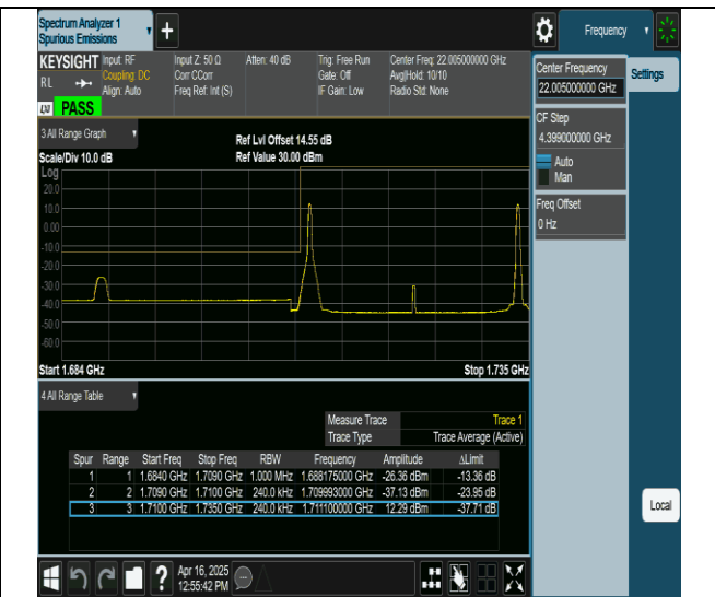
66-66-20MHz-5MHz-QPSK@QPSK-QPSK@QPSK-132072-132189-1RB#0@0RB#0-1RB#24@0RB#0-PASS
