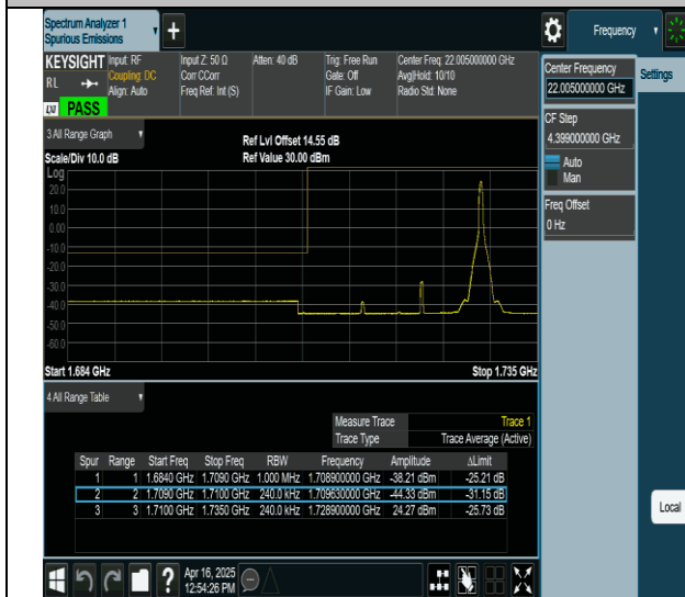
66-66-20MHz-5MHz-QPSK@QPSK-QPSK@QPSK-132072-132189-1RB#99@0RB#0-0RB#0@0RB#0-PASS
