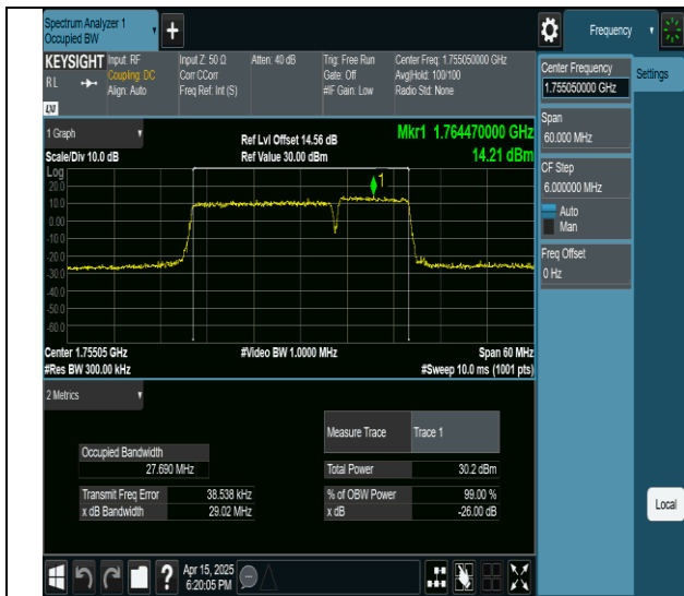
66-66-20MHz-10MHz-QPSK-QPSK-132373-132517-100RB#0-50RB#0-PASS
