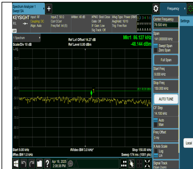
66-66-20MHz-20MHz-QPSK-QPSK-132374-132572-1RB#0- ORB#0-0.009~0.15MHz-PASS
