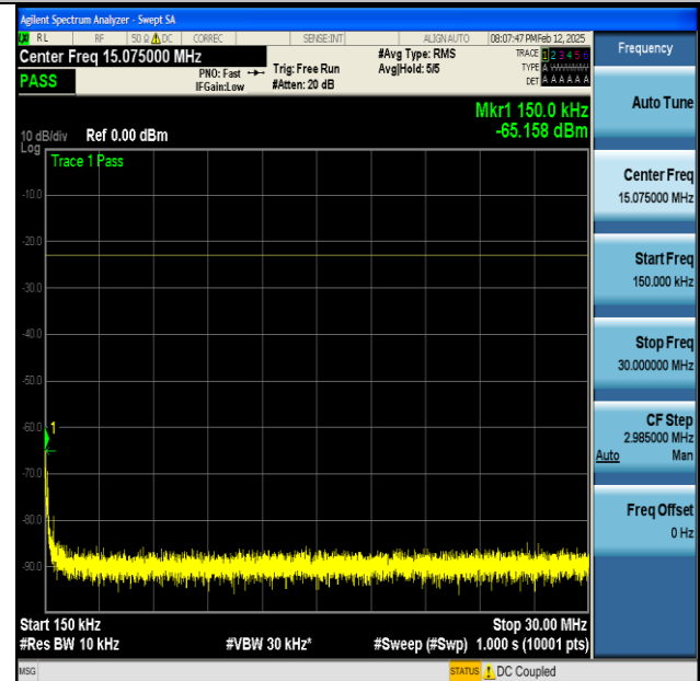
NTNV-n71-PC3-15-20-L-CP-QPSK-Edge_1RB_Left-0.15- 30-PASS
