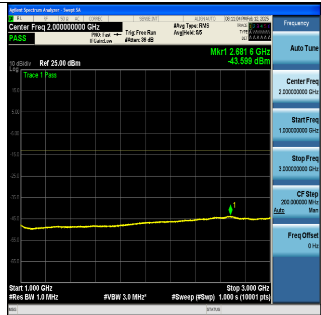
NTNV-n71-PC3-15-20-M-CP-QPSK-Edge_1RB_Left-1000-3000-PASS
