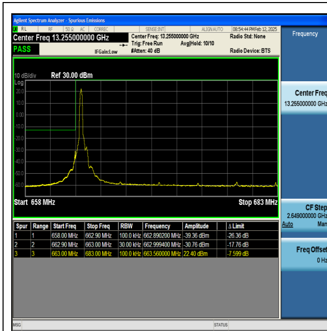
NTNV-n71-PC3-15-20-L-DFT-BPSK-Edge_1RB_Left-PASS
