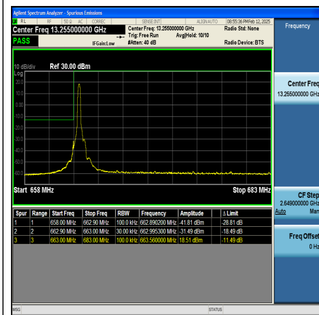
NTNV-n71-PC3-15-20-L-CP-QPSK-Edge_1RB_Left-PASS
