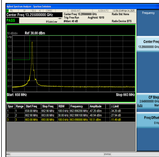
NTNV-n71-PC3-15-30-L-CP-QPSK-Edge_1RB_Left-PASS
