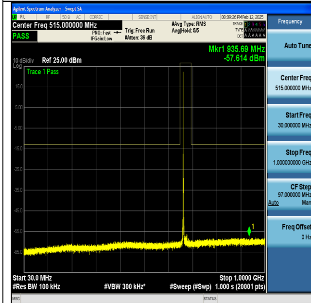
NTNV-n71-PC3-15-20-M-DFT-BPSK-Edge_1RB_Left-30- 1000-PASS
