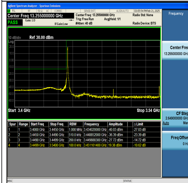
NTNV-n77(3450-3550)-PC2-30-90-L-CP-QPSK- Edge_1RB_Left-PASS
