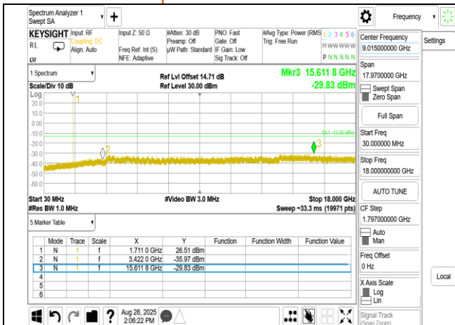
Band4 15MHz Chain0 1717.5MHz NBI 0 QPSK 1 0
