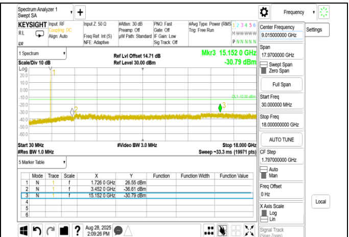
Band4 15MHz Chain0 1732.5MHz NBI 0 QPSK 1 0
