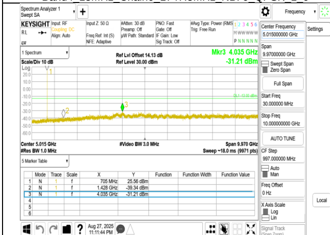
Band12 5MHz Chain0 707.5MHz NBI 0 QPSK 1 0
