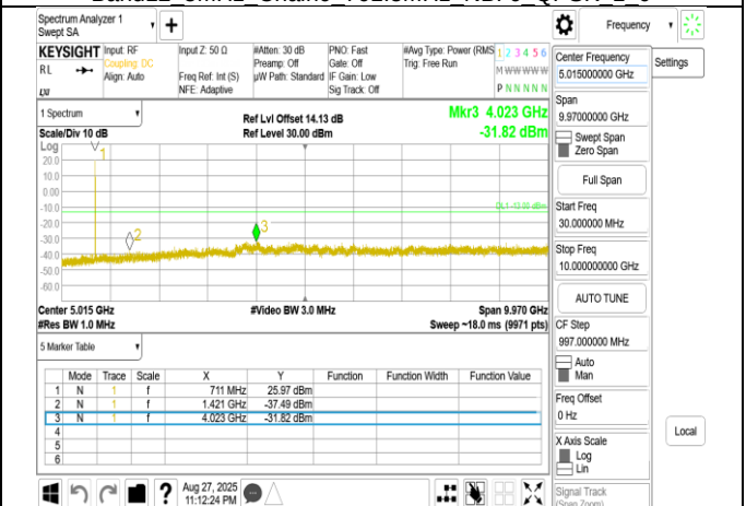
Band12 5MHz Chain0 713.5MHz NBI 0 QPSK 1 0
