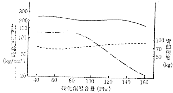
圖 II 2.2 硬化劑混合量和粘附強度 (在80°C一小時的硬化) 試驗片：以及其他同圖 II 2.1
