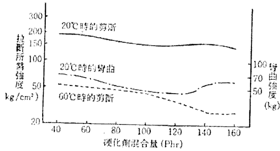
圖 II 2.1 硬化劑混合量和粘附強度 (在20°C七天的硬化) 試驗片：軟鋼板 (25×100×1.6mm) (Over-lap)12.5mm
