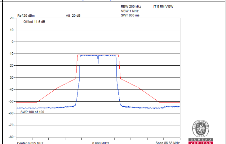
802.11be (EHT20) / Chain 3 : CH 181
