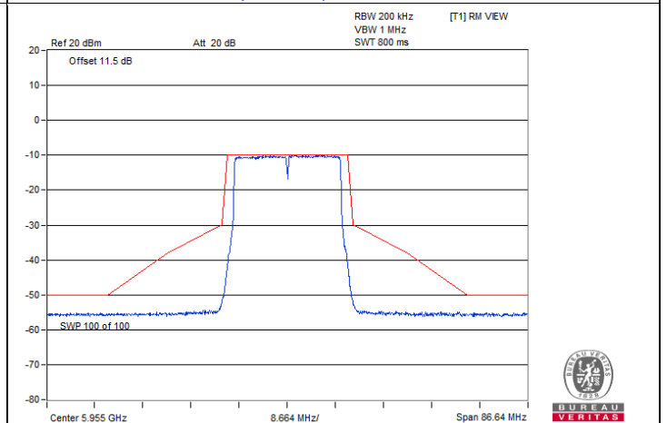
802.11be (EHT20) / Chain 3 : CH 1
