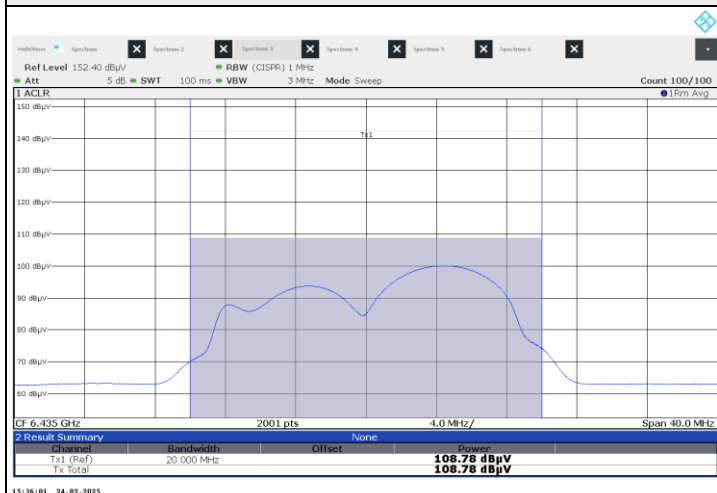
802.11a CDD : CH 97
