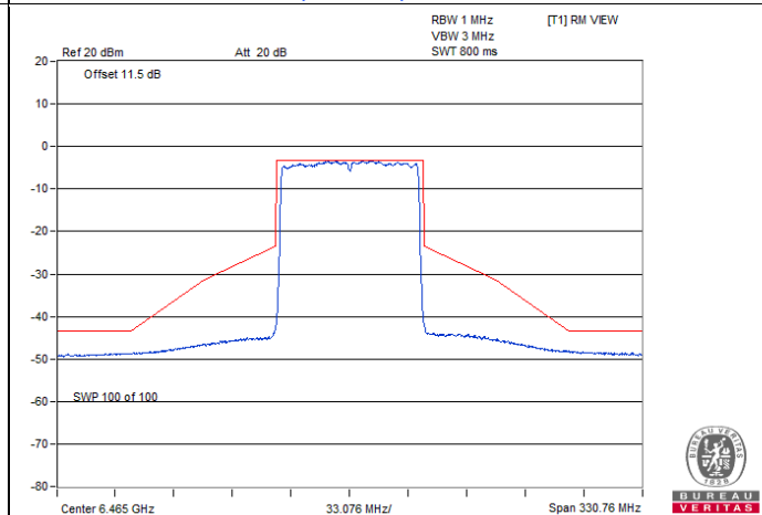
802.11be (EHT80) / Chain 2 : CH 103
