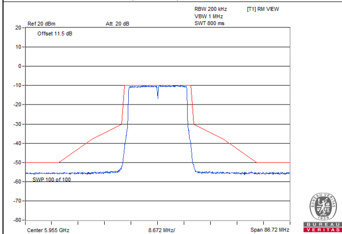
802.11be (EHT20) / Chain 2 : CH 1
