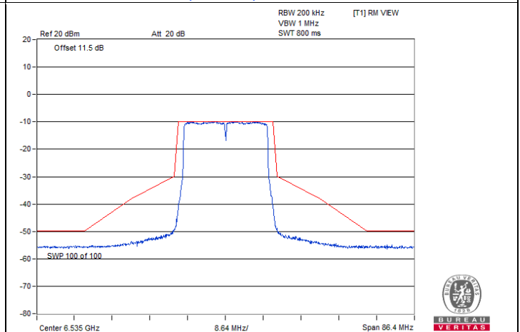
802.11be (EHT20) / Chain 3 : CH 117
