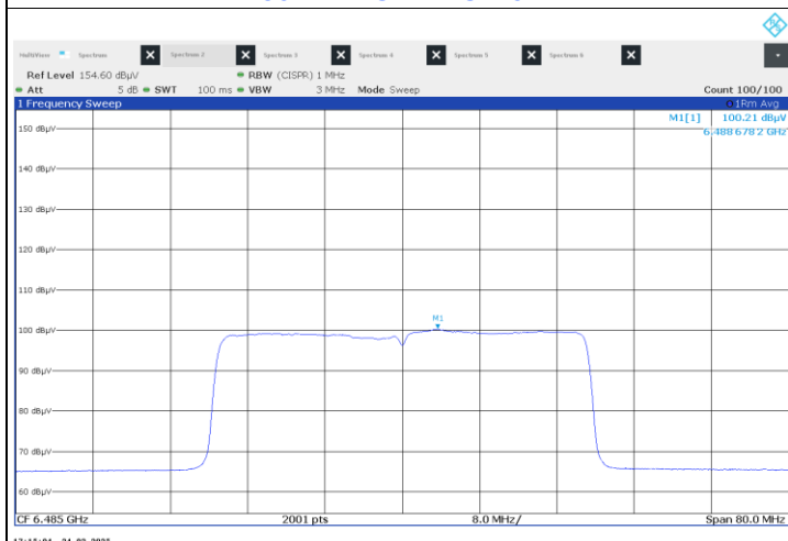
802.11be (EHT40) Beamforming : CH 107
