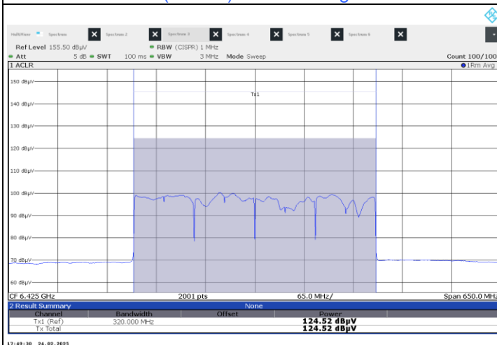
802.11be (EHT320) Beamforming : CH 95
