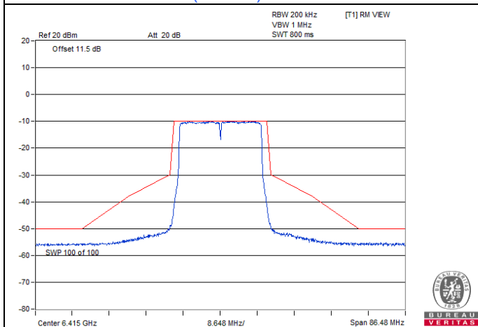
802.11be (EHT20) / Chain 2 : CH 93
