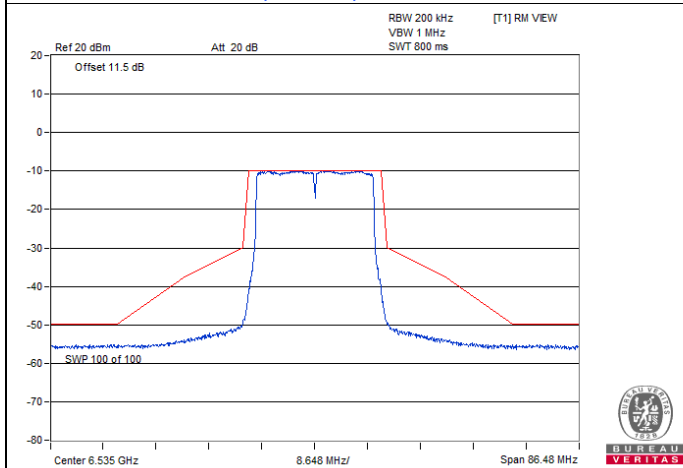
802.11be (EHT20) / Chain 2 : CH 117
