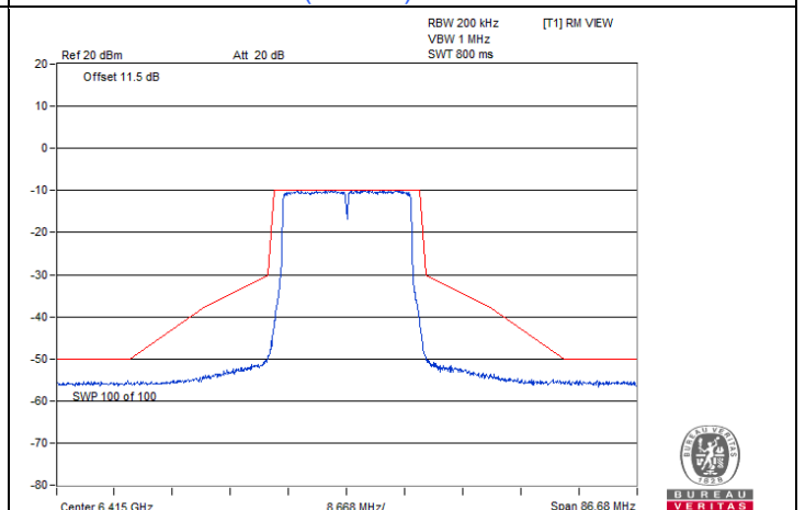
802.11be (EHT20) / Chain 3 : CH 93
