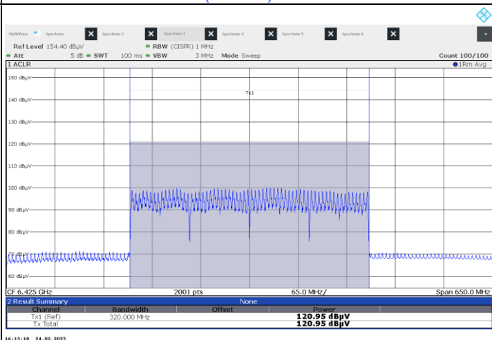
802.11be (EHT320) CDD : CH 95
