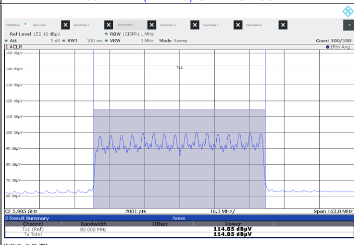
802.11be (EHT80) CDD : CH 7
