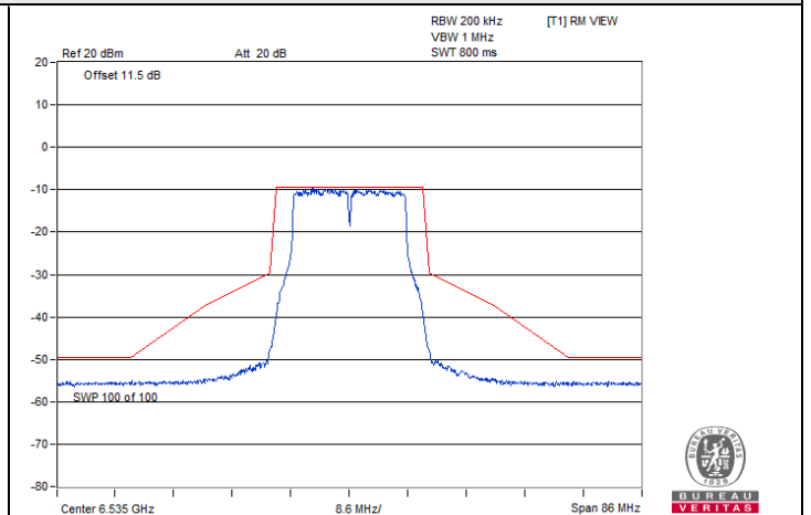
802.11a / Chain 1 : CH 117
