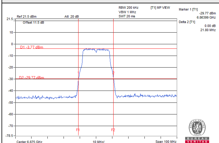
802.11a / Chain 2 : CH 185
