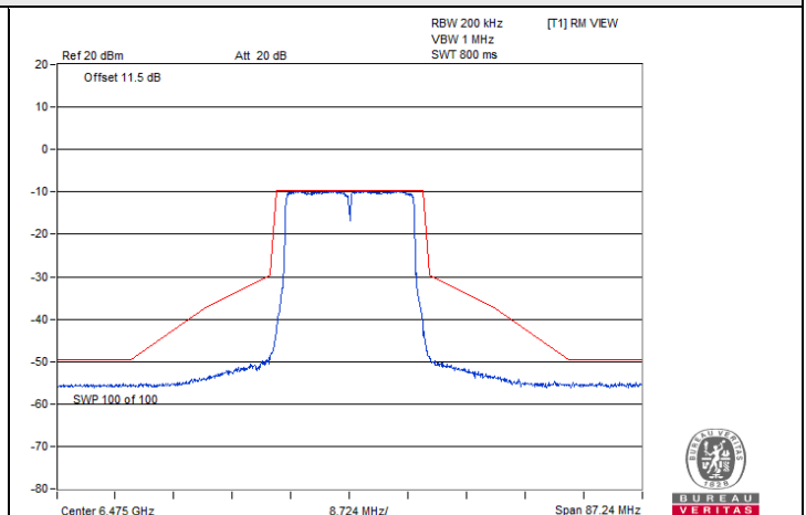
802.11be (EHT20) / Chain 3 : CH 105
