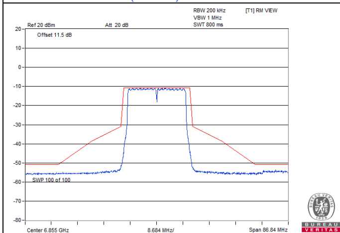
802.11be (EHT20) / Chain 2 : CH 181
