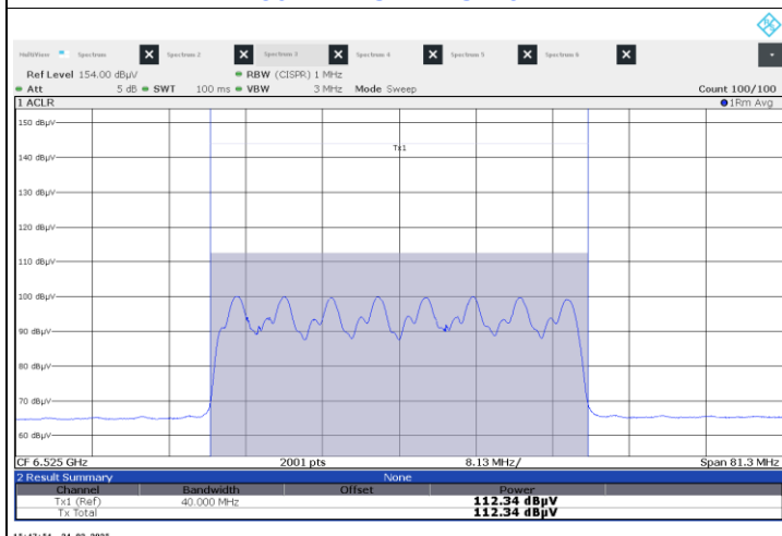
802.11be (EHT40) CDD : CH 115
