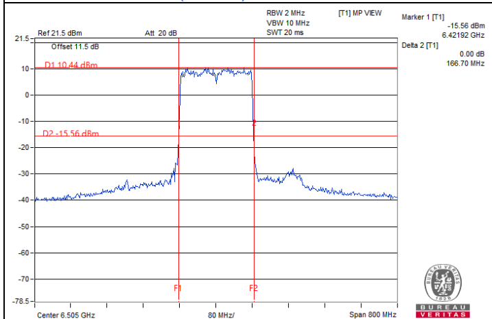
802.11be (EHT160) / Chain 3 : CH 111
