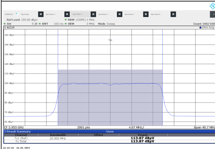
802.11be (EHT20) Beamforming : CH 1
