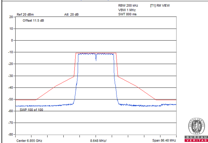
802.11be (EHT20) / Chain 0 : CH 181
