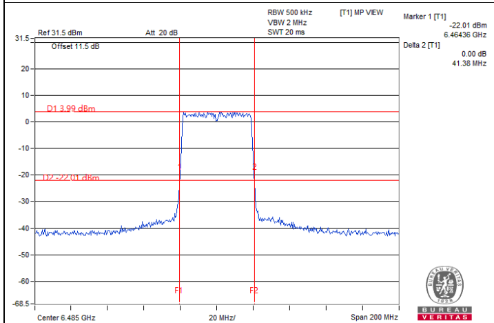
802.11be (EHT40) / Chain 0 : CH 107
