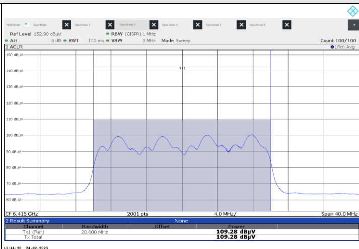
802.11be (EHT20) CDD : CH 93
