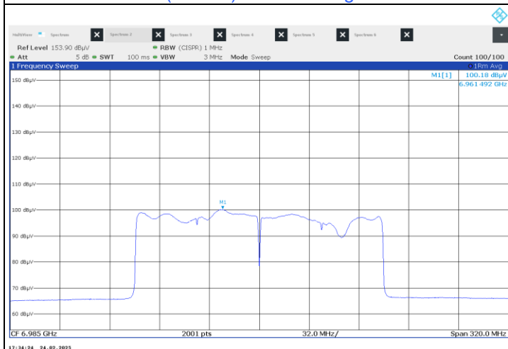
802.11be (EHT160) Beamforming : CH 207
