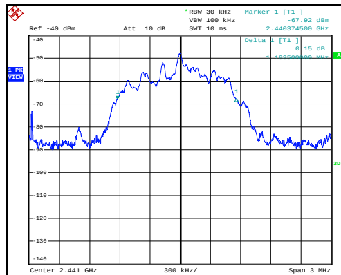
Figure 7.3.2-8: 20dB BW Mid CH ( \pi/4 DQPSK - 2Mbps)
