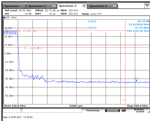
Figure 7.4.1.2-8: Upper Band-Edge Hopping - OOK
