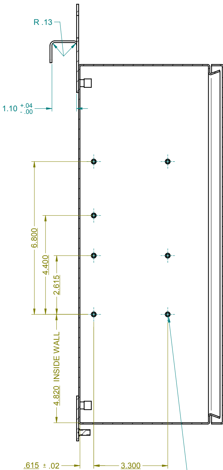
SECTION A-A
