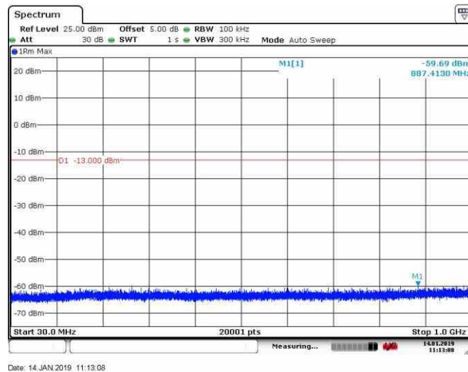
Band4_20MHz_QPSK_20175_1RB#0
