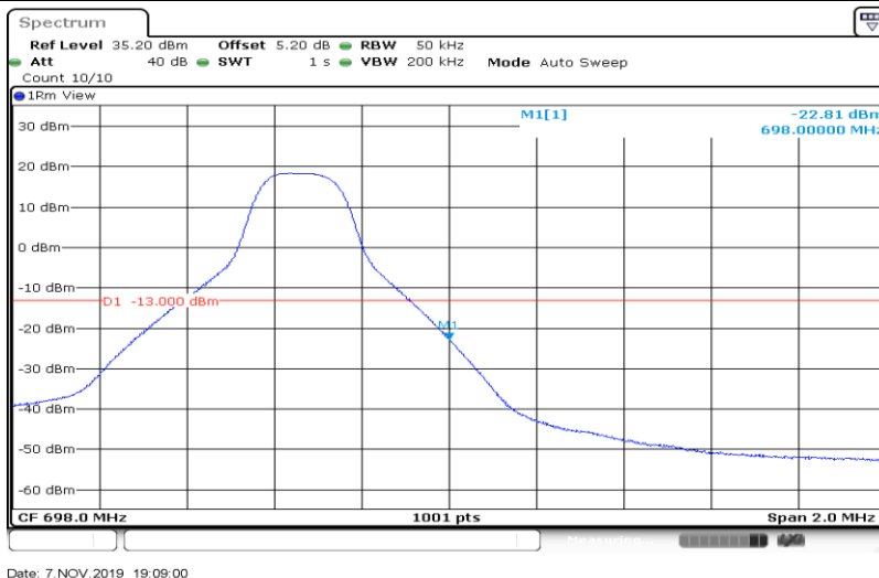
Band71-5MHz-QPSK-133447-25RB#0
