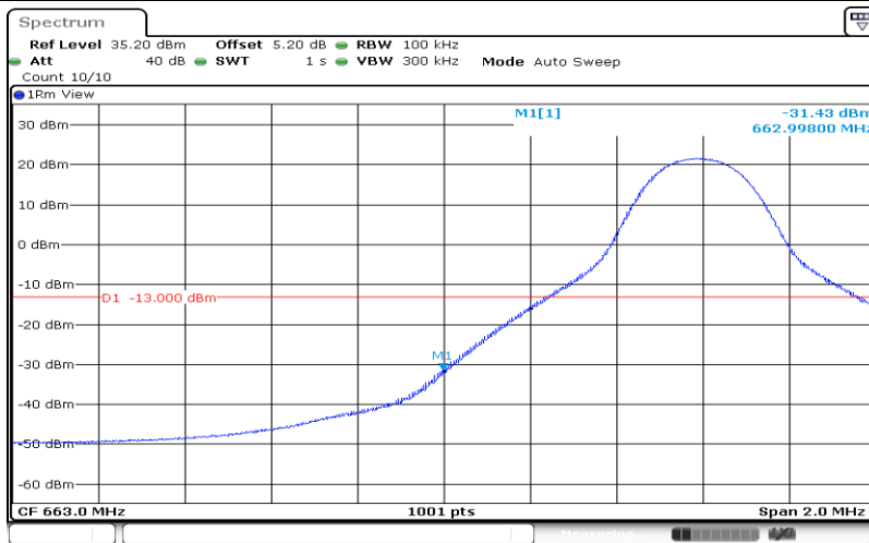
Band71-10MHz-QPSK-133172-50RB#0
