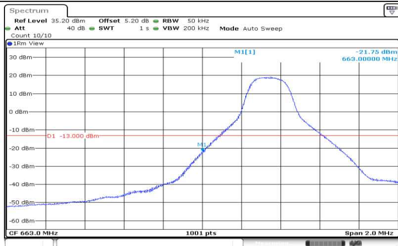
Band71-5MHz-QPSK-133147-1RB#0
