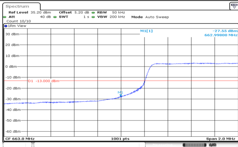
Band71-5MHz-QPSK-133147-25RB#0
