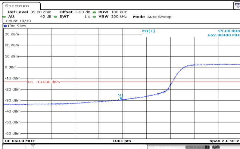
Band71-10MHz-QPSK-133172-50RB#0
