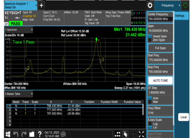
Band Edge Band13 10MHz QPSK RB50 0 CH23230
