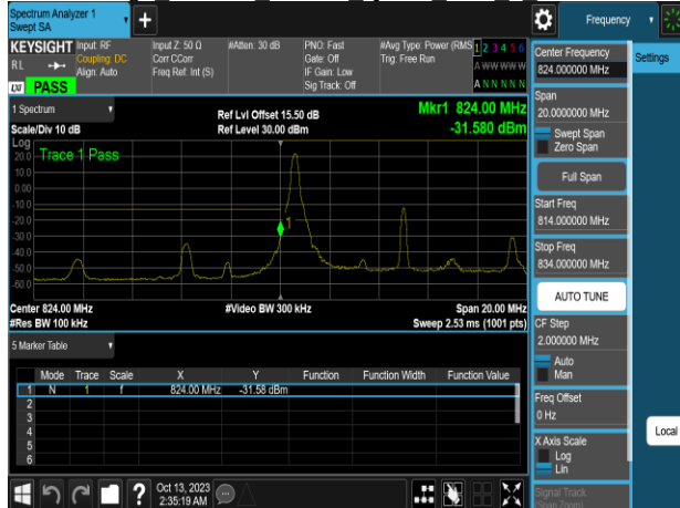
Band Edge Band26 10MHz QPSK RB1 49 CH26990
