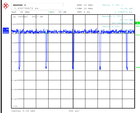
802.11a
