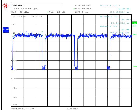
802.11n HT40
