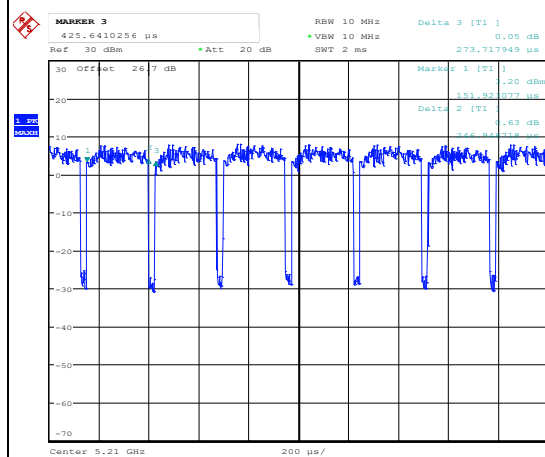
802.11ac VHT80
