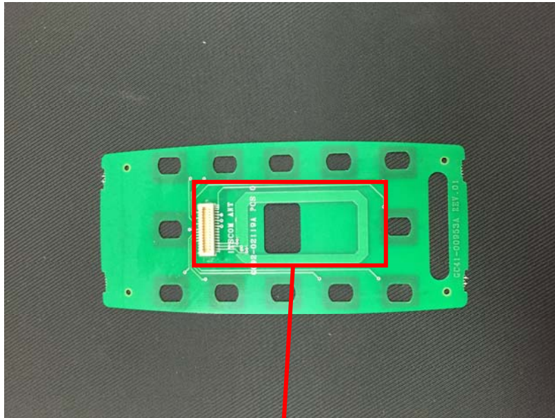
RFID(13.56 MHz) Antenna
