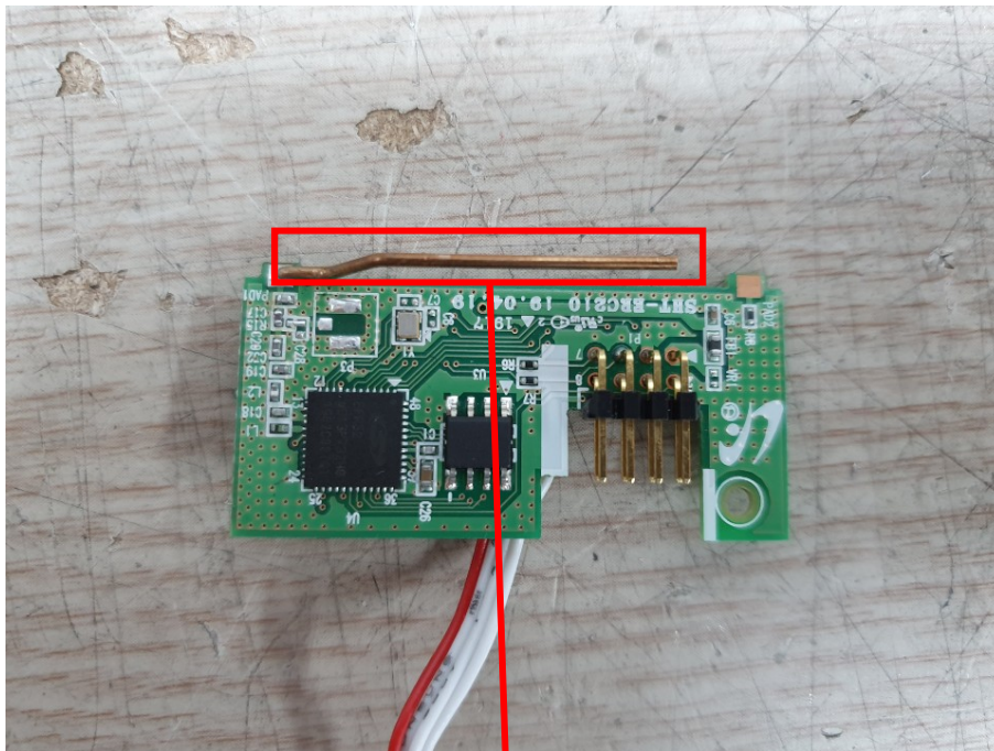
RFID(13.56 MHz) Antenna
