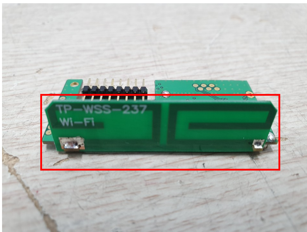
Antenna_WiFi 2.4 GHz
