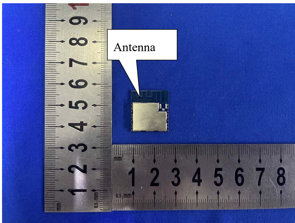
Photo 3:WIFI/BLE Antenna
