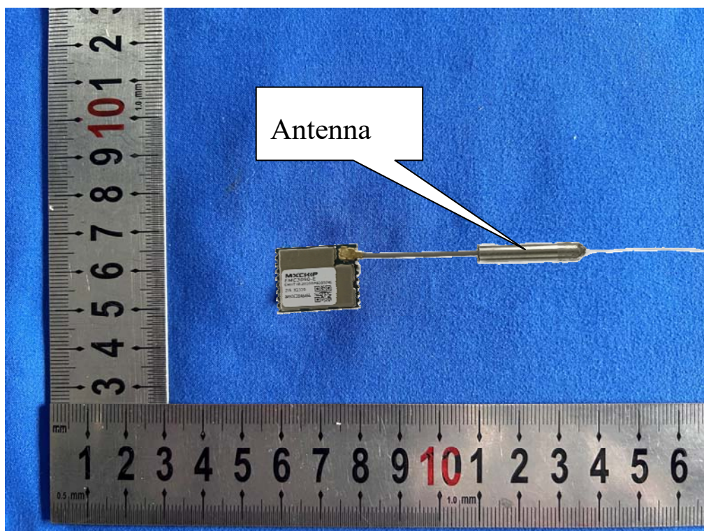
Photo 3:WIFI/BLE Antenna
