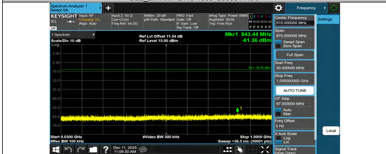
BLE_2M-Ant1-2478-30~1000-PASS
