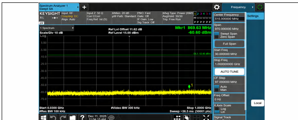
BLE_2M-Ant1-2404-30~1000-PASS
