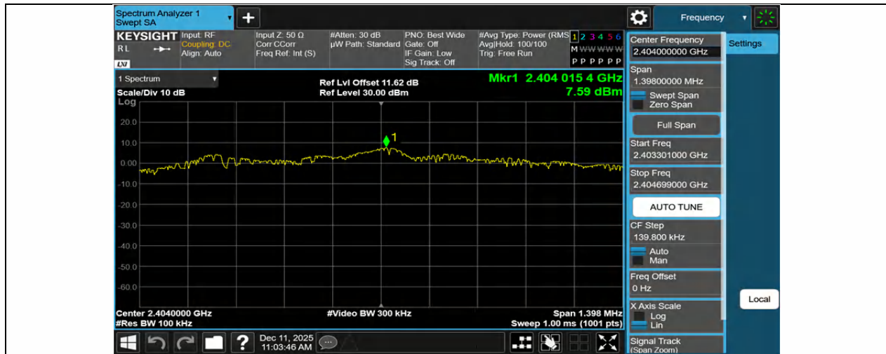
BLE 2M-Ant1-2404-PASS
