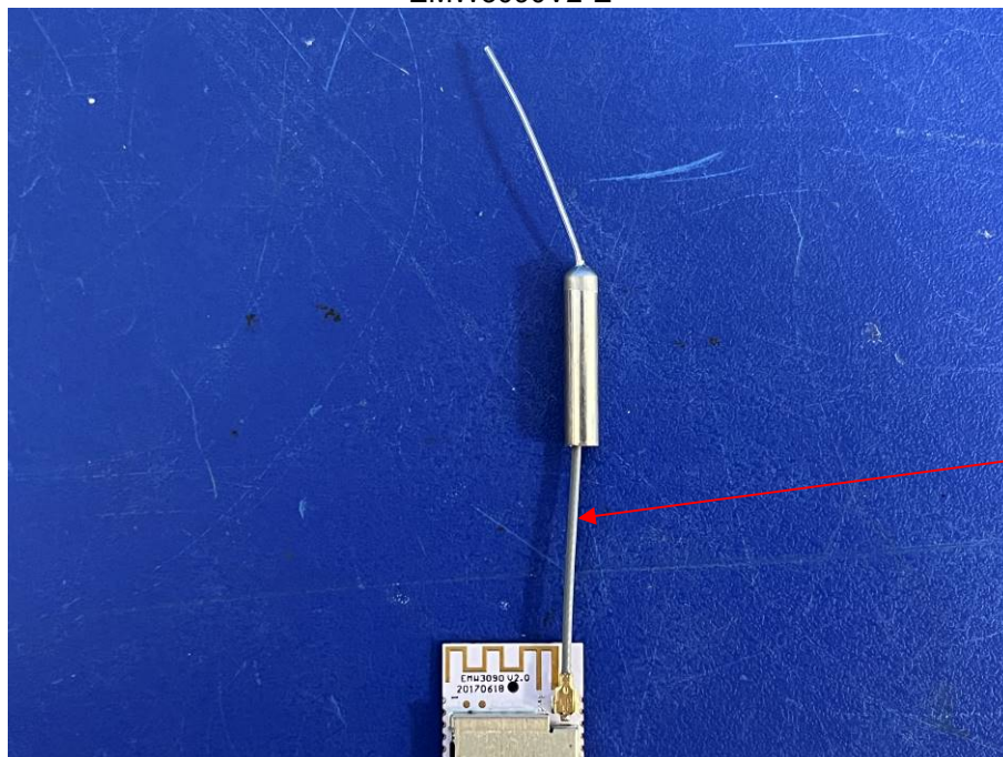
EMW3090V2-E
