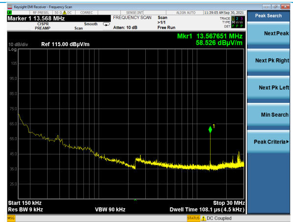
Perpendicular: 0.15 – 30 MHz
