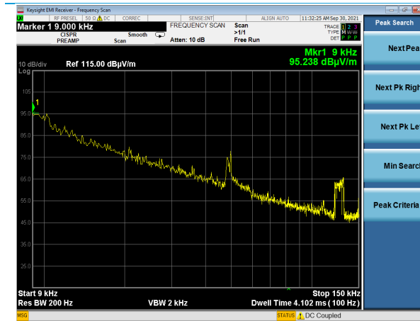
Perpendicular: 9 – 150 kHz
