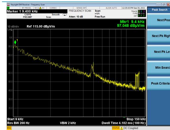
Parallel: 9 – 150 kHz
