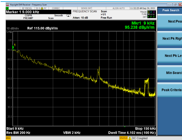
Perpendicular: 9 – 150 kHz
