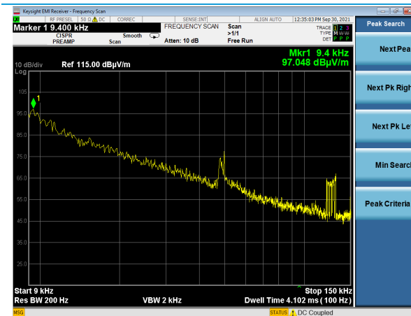
Parallel: 9 – 150 kHz
