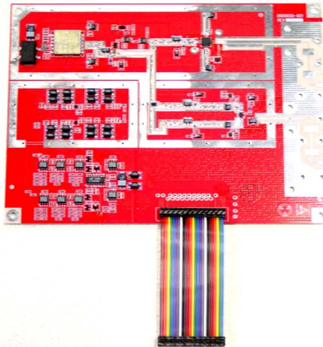
RF PCA Top
