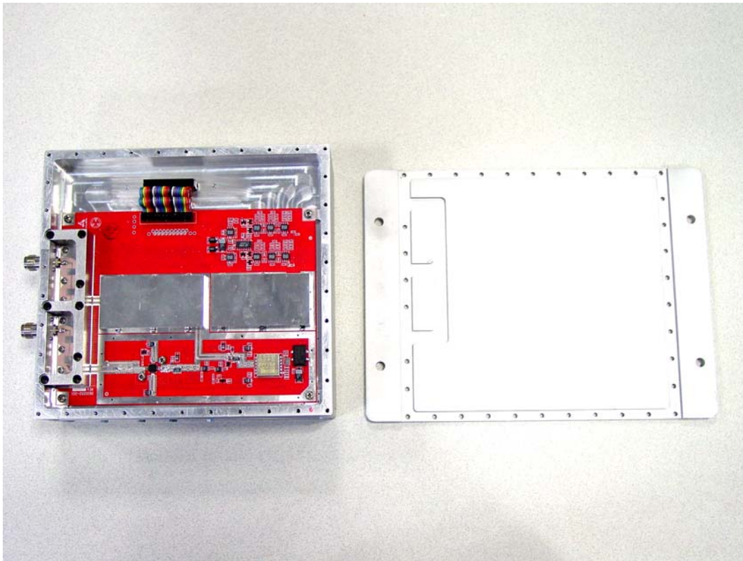
B2450R01-A Assembly RF
