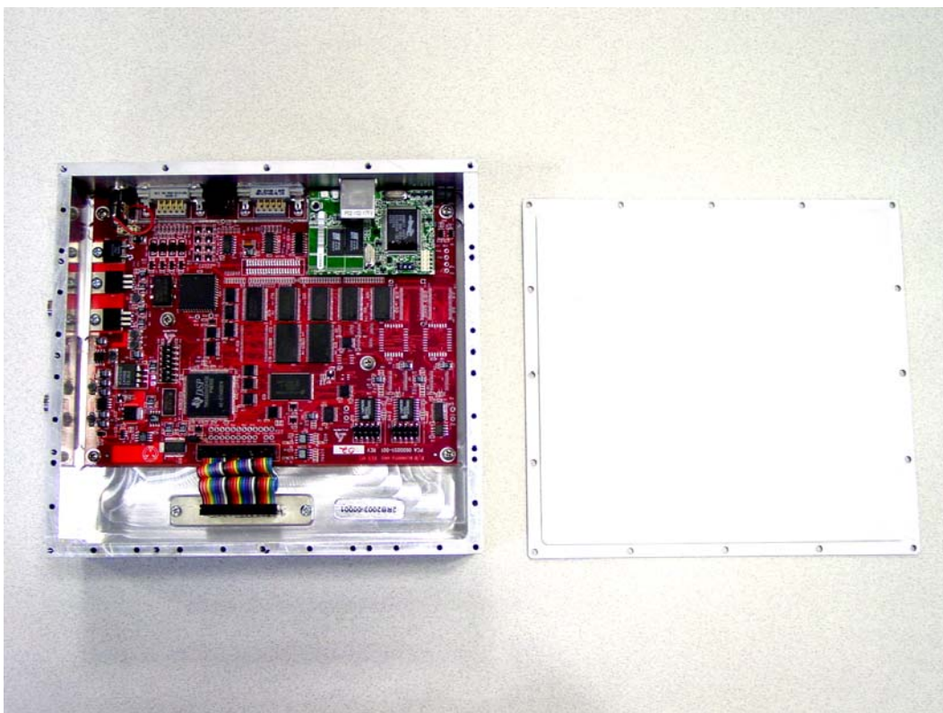
B2450R01-A Assembly Digital
