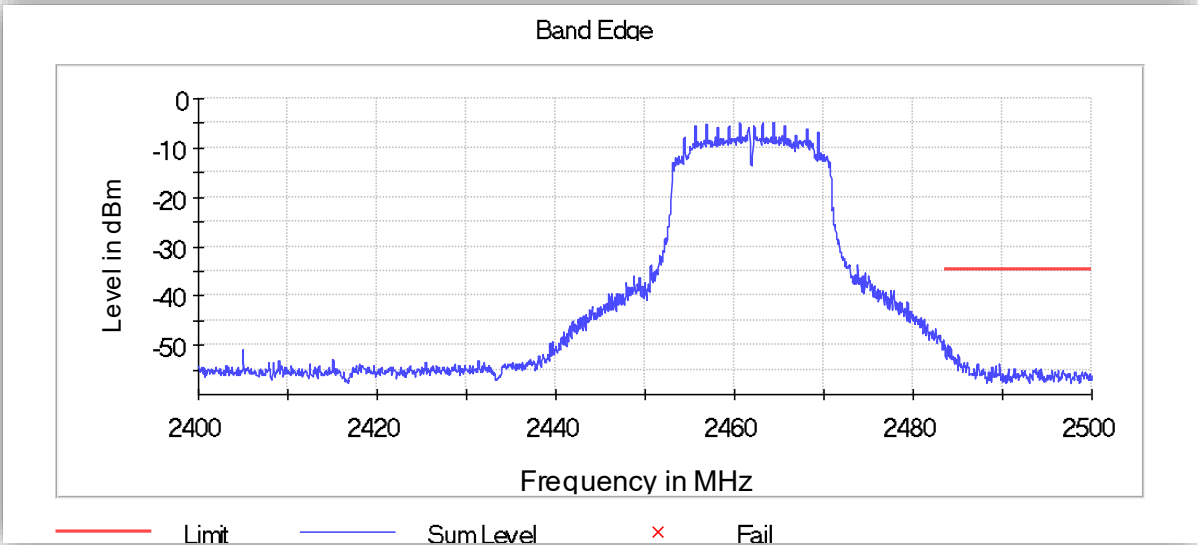
WLAN 802.11n MCS0 Upper Band Edge 2483.5MHz
