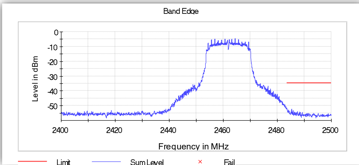
WLAN 802.11g 6Mbps Upper Band Edge 2483.5MHz
