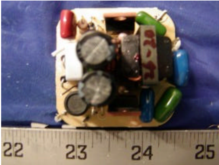
EUT - Component View (RPW-26E)
